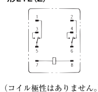
端子配置/内部接続図 (BOTTOM VIEW) 形LY2 (Z) 形LY2 (Z)-D
