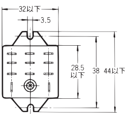
取り付け穴加工寸法
