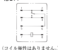
端子配置/内部接続図 (BOTTOM VIEW) 形LY1 形LY1N-D
