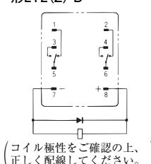
端子配置/内部接続図 (BOTTOM VIEW) 形LY2 (Z) 形LY2 (Z)-D
