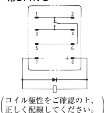
端子配置/内部接続図 (BOTTOM VIEW) 形LY1 形LY1N-D
