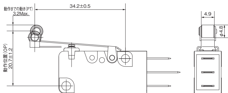
外形寸法図
