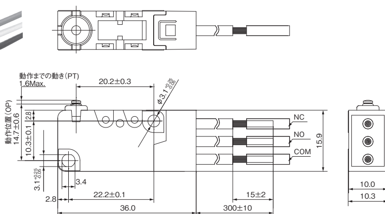
外形寸法図
