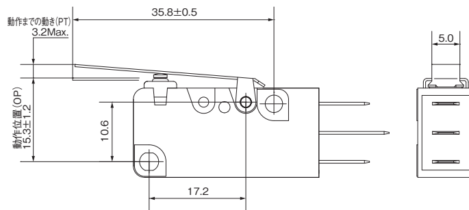
外形寸法図
