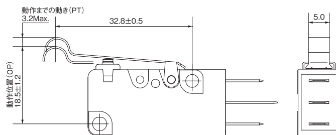
外形寸法図
