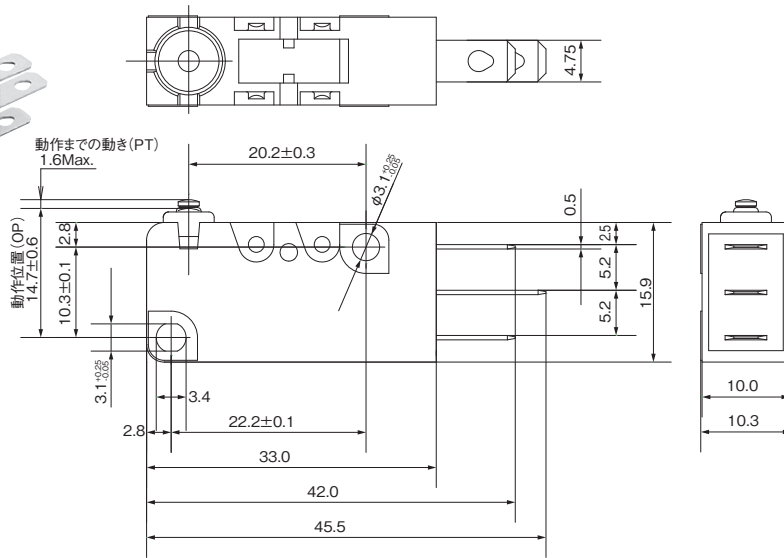
外形寸法図
