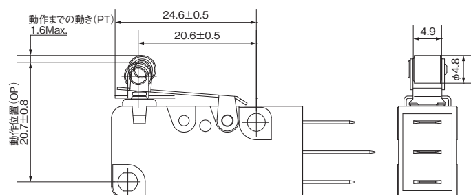
外形寸法図
