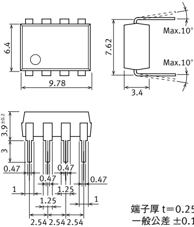
標準P/C板端子 外形寸法図
