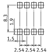
実装パッド(TOP VIEW)
