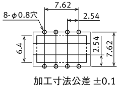
実装パッド(TOP VIEW)
