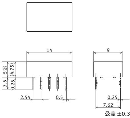
プリント板端子 (自立端子)
