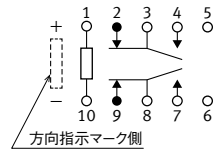
内部結線図 (BOTTOM VIEW) シングルスティプル型 (無励磁状態)
