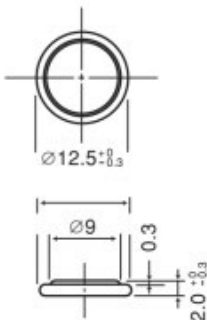
外形寸法図
