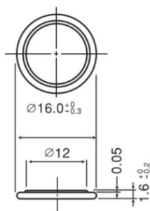
外形寸法図
