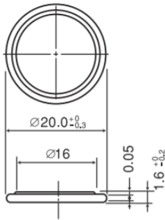
外形寸法図
