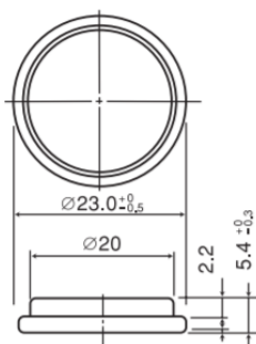
外形寸法図
