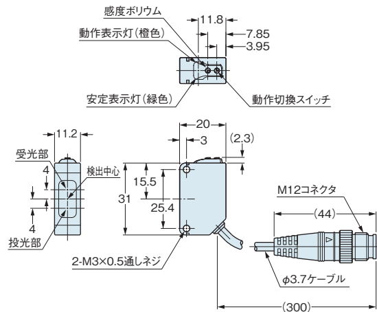
CX-49□-J CX-48□-J CX-42□-J
