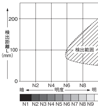
明度-検出距離特性
