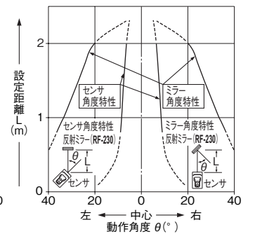
角度特性
