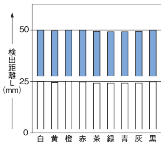
色(50×50mm色画用紙)-検出距離特性
