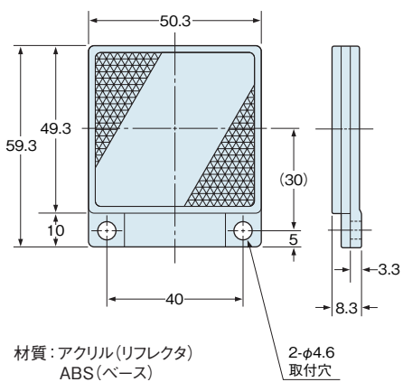
RF-230 反射ミラー(ベーシックタイプを除くミラー反射型に付属)
