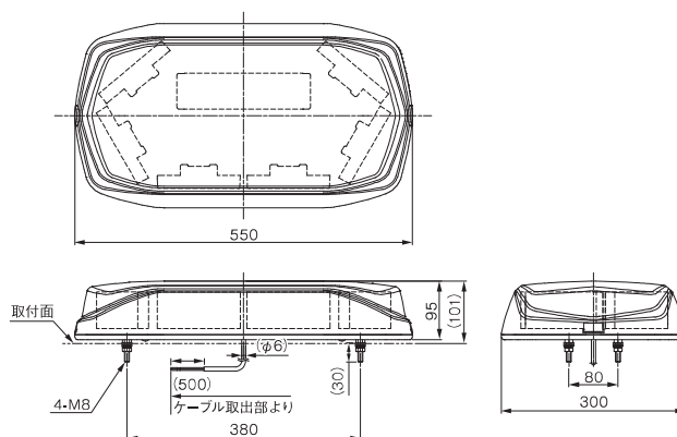
外観図 (単位: mm)
