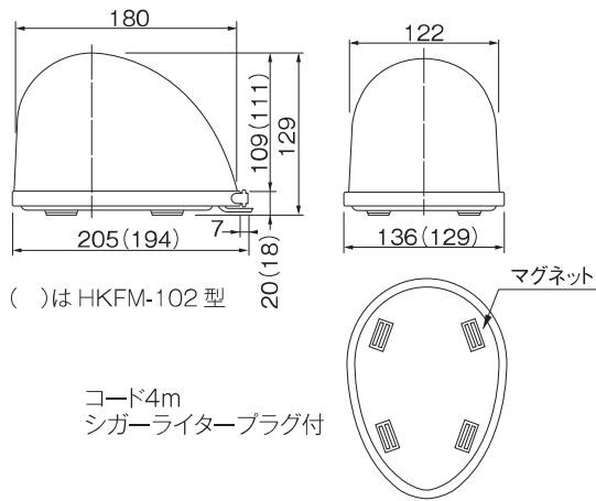
外観図 (単位: mm)
