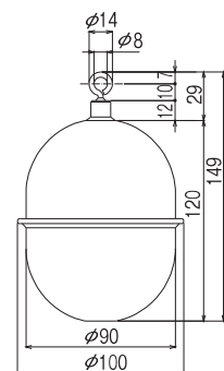
TBLC108S (上限警報用ステンレス錘)
