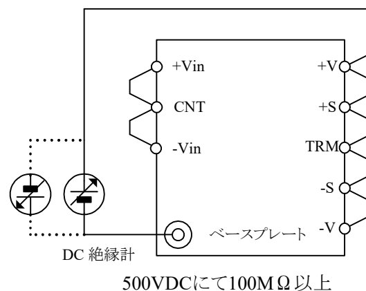
図7-31 絶縁抵抗試験方法
