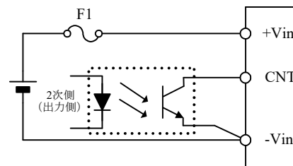
図7-19 CNT接続例(2)
