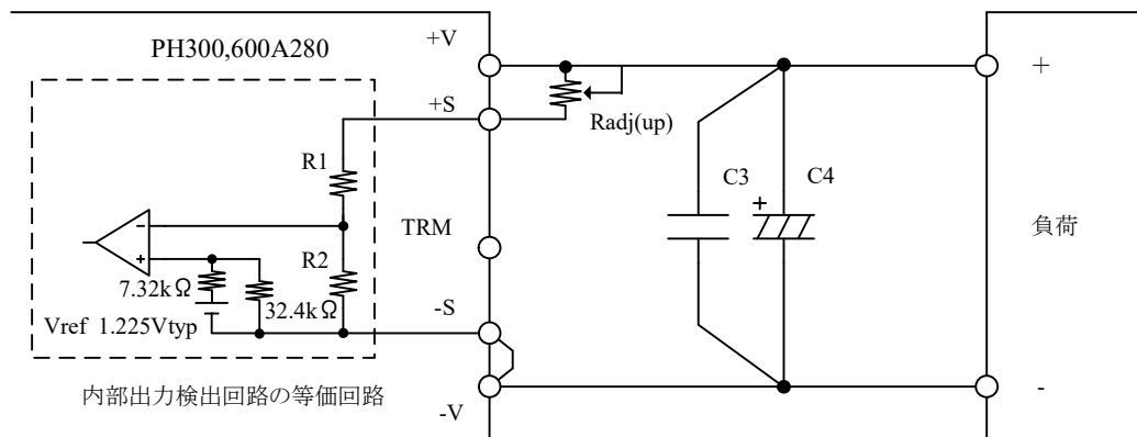
図7-9 外付け抵抗の接続例 (出力電圧を高く設定する場合)
