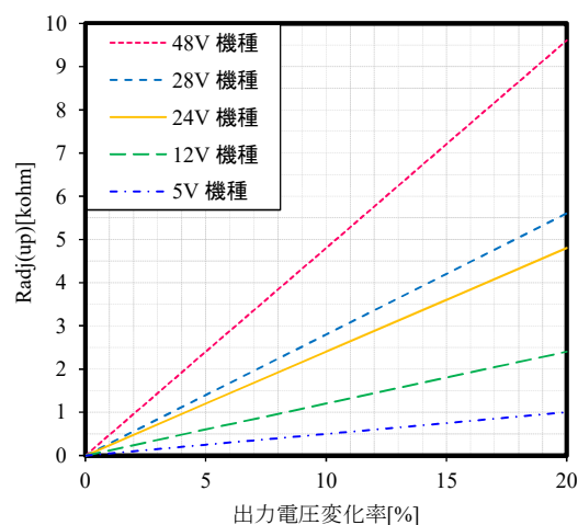
図7-10 外付け抵抗(Radj(up)) 対 Δ(%)
