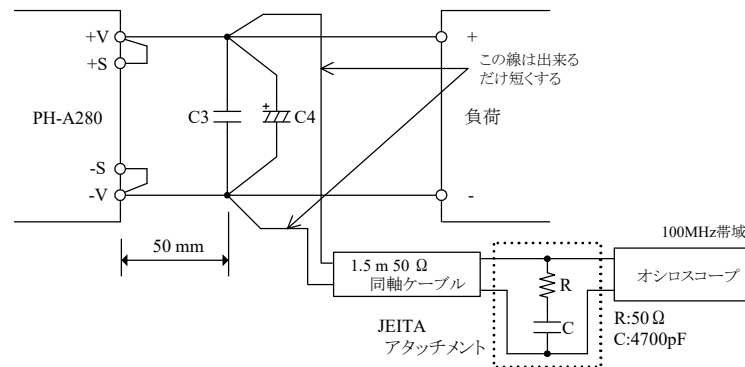
図7-15 出力リップル電圧(含スパイクノイズ)測定方法
