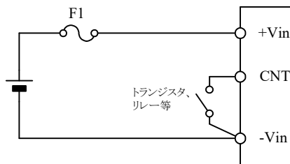
図7-18 CNT接続例(1)
