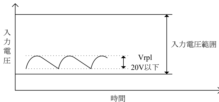
図7-1 入力リップル電圧
