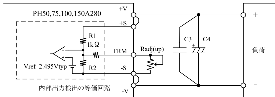
図7-7 外付け抵抗の接続例 (出力電圧を高く設定する場合)
