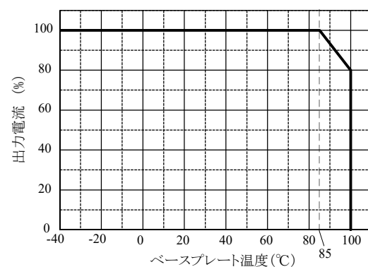
図7-26 ディレーティングカーブ
