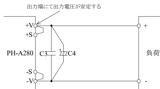
図7-17 リモートセンシングしない場合 (ローカルセンシング)
