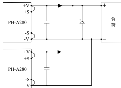
図7-21 冗長運転接続方法
