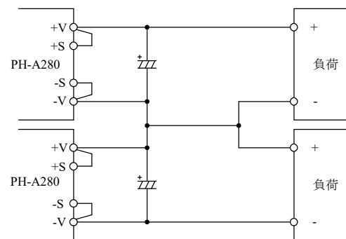
図7-23 ±出力使用の直列運転
