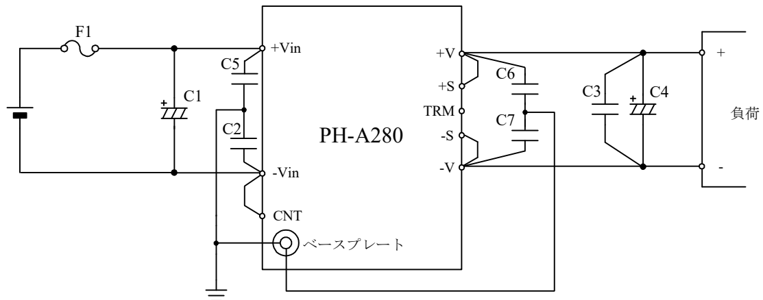
図6-1 基本的な接続
