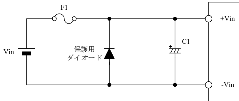
図6-2 入力の逆接続保護
