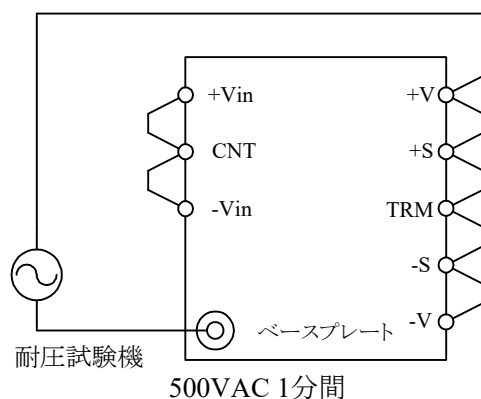
図7-29 出力 - ベースプレート間耐電圧試験方法
