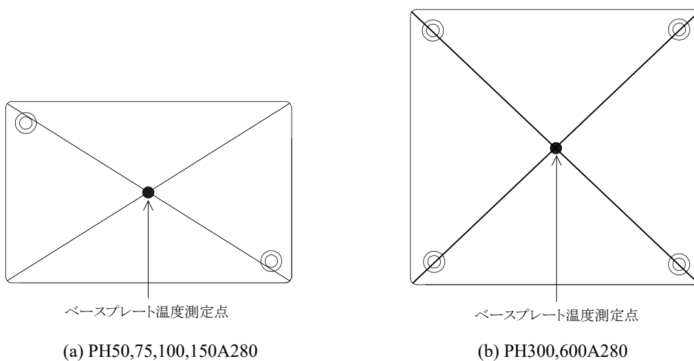
図7-24 ベースプレート温度測定点
