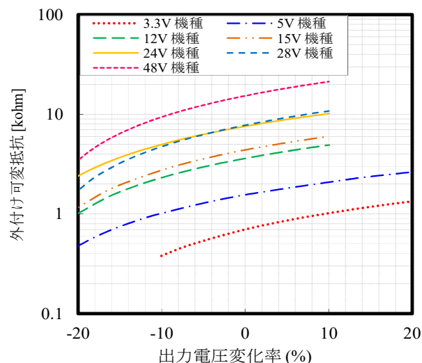
図7-12 外付け可変抵抗(VR) 対 Δ(%)
