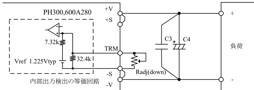
図7-5 外付け抵抗の接続例 (出力電圧を低く設定する場合)
