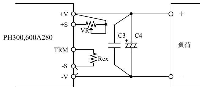
図7-13 外付け抵抗の接続例 (可変範囲内で出力電圧を調整する場合)
