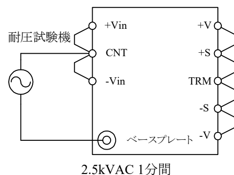
図7-28 入力 - ベースプレート間耐電圧試験方法
