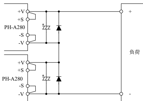
図7-22 出力電圧積み重ね直列運転
