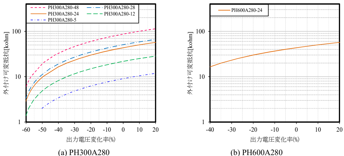
図7-14 外付け可変抵抗(VR) 対 Δ(%)
