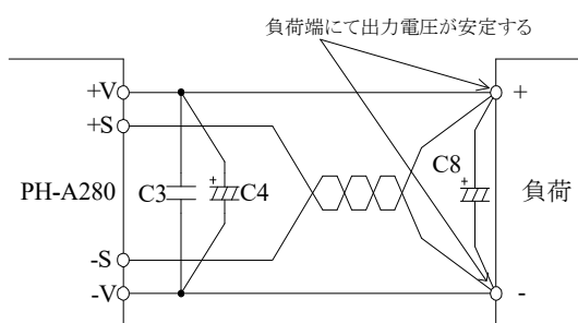
図7-16 リモートセンシングする場合
