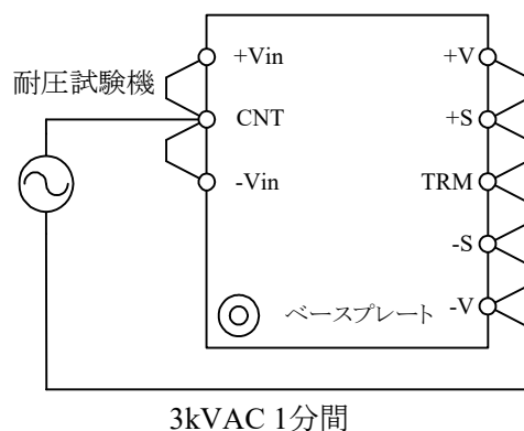
図7-27 入力 - 出力間耐電圧試験方法
