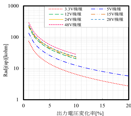
図7-8 外付け抵抗(R adj(up) ) 対 Δ(%)
