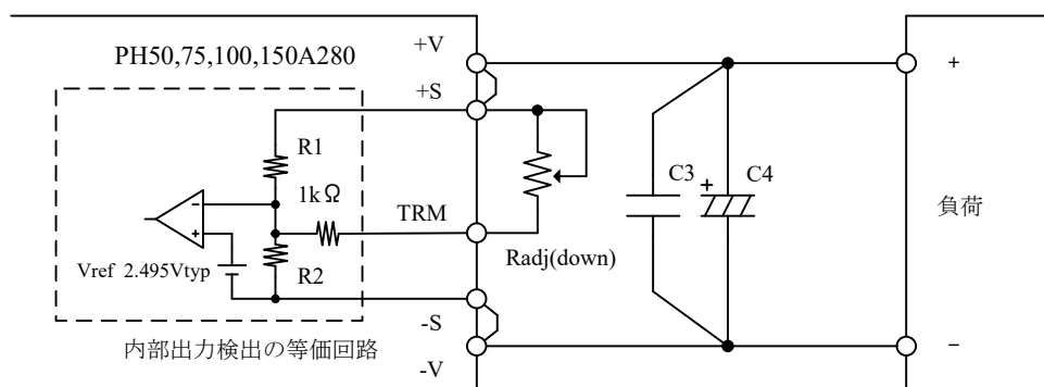
図7-3 外付け抵抗の接続例 (出力電圧を低く設定する場合)
