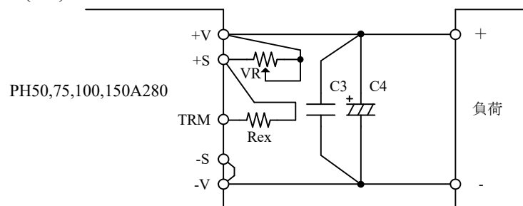
図7-11 外付け抵抗の接続例 (可変範囲内で出力電圧を調整する場合)
