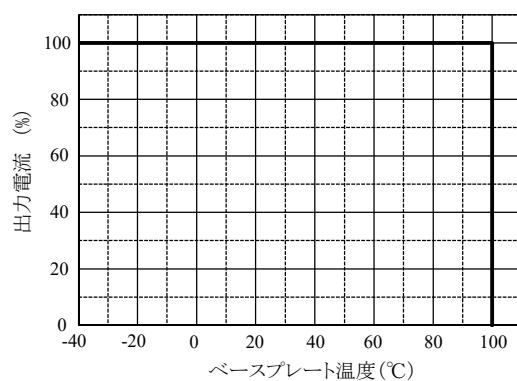
図7-25 ディレーティングカーブ
