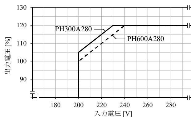
図7-2 入力電圧の制限
