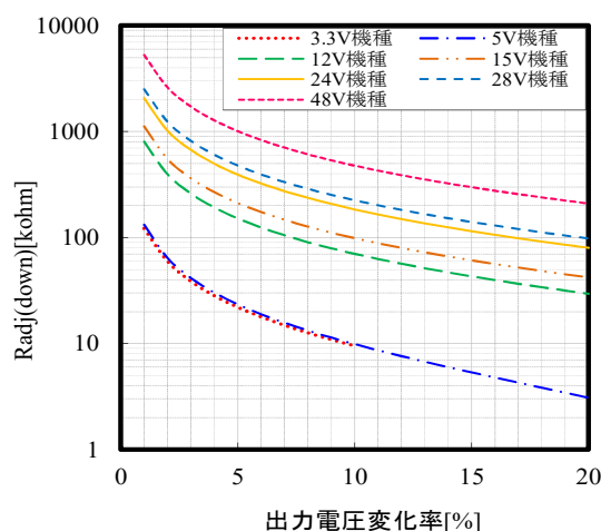
図7-4 外付け抵抗(Radj(down)) 対 Δ(%)
