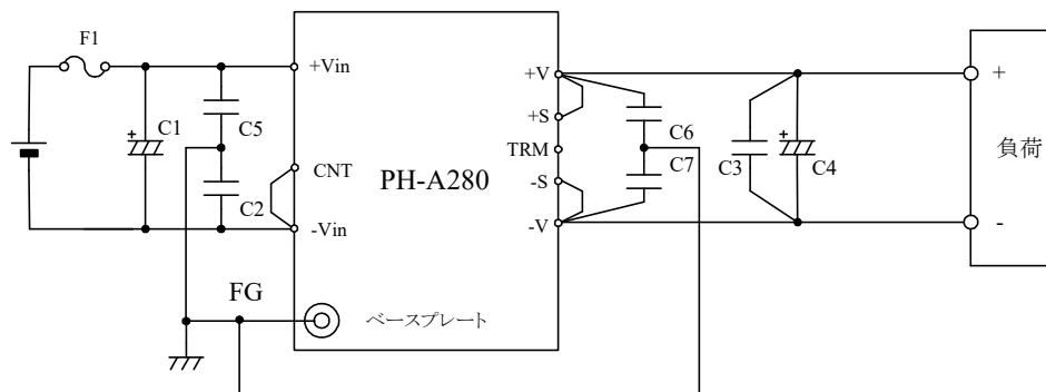
図7-30 外付け部品接続例
