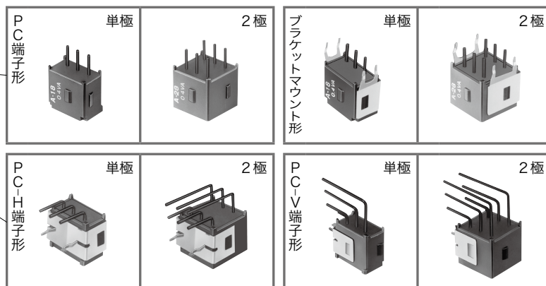
端子部形状
