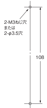
取り付け穴加工寸法
