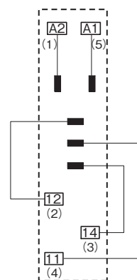
端子配置/内部接続図 (TOP VIEW)
