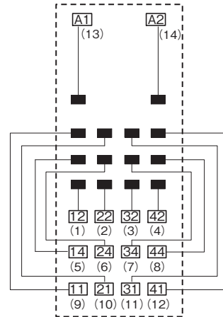
端子配置/内部接続図 (TOP VIEW)
