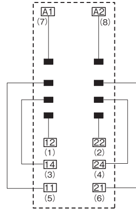
端子配置/内部接続図 (TOP VIEW)
