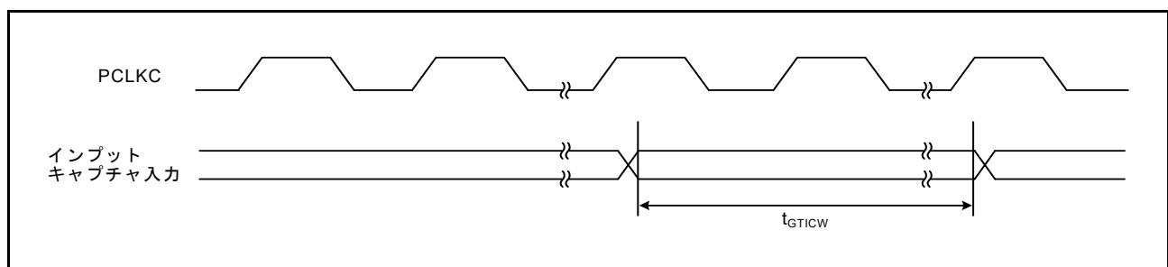
図2.46 GPTa インプットキャプチャ入力タイミング
