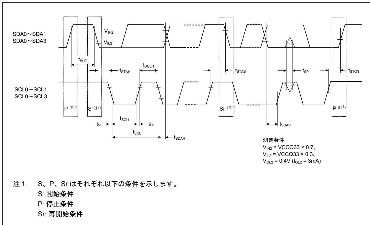
図 2.64 RIICa バスインタフェース入出力タイミング
