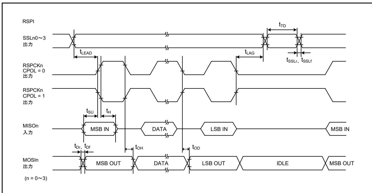
図 2.53 RSPiA タイミング (マスタ、CPHA = 0)
