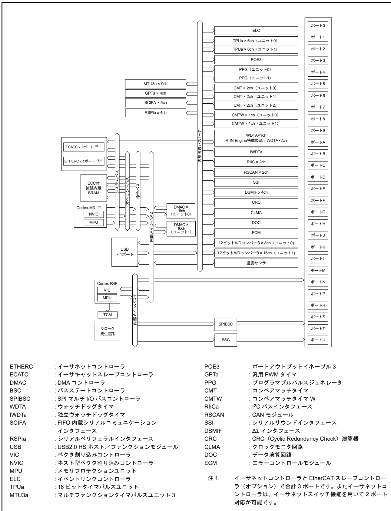
図 1.1 ブロック図
