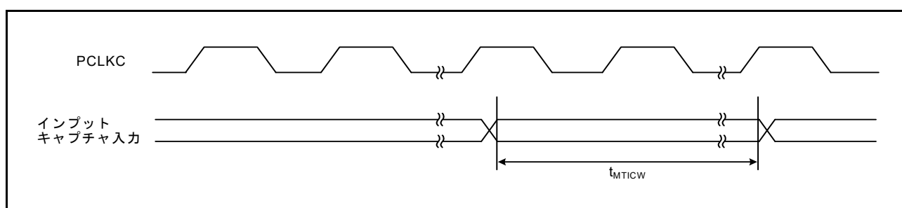
図 2.43 MTU3a インพุットキャプチャ入力タイミング
