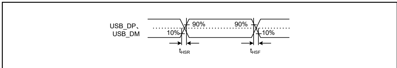
図 2.84 USB_DP、USB_DM 出力タイミング (ハイスピード時)
