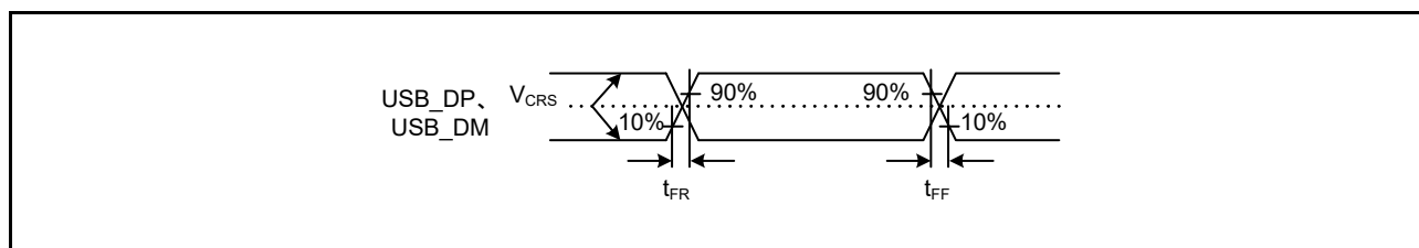
図 2.82 USB_DP、USB_DM 出力タイミング (フルスピード時)
