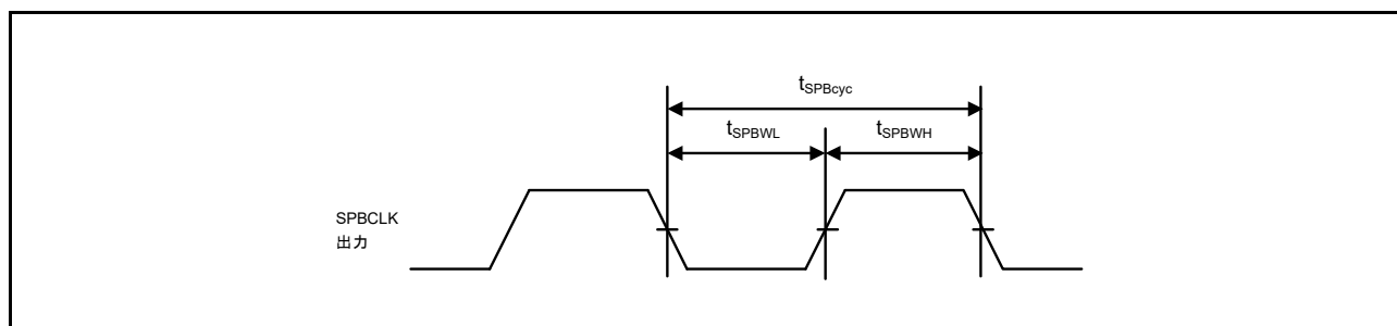
図 2.57 SPIBSC クロックタイミング
