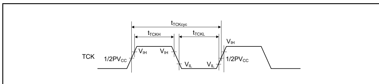
図 2.87 TCK 入力タイミング
