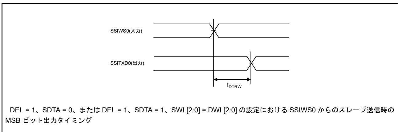
図 2.68 SSIWS0 変化エッジからの SSITXD0 出力遅延
