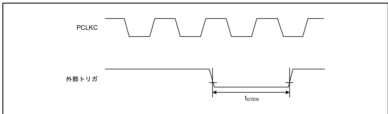
図2.47 GPTa 外部トリガ入力タイミング
