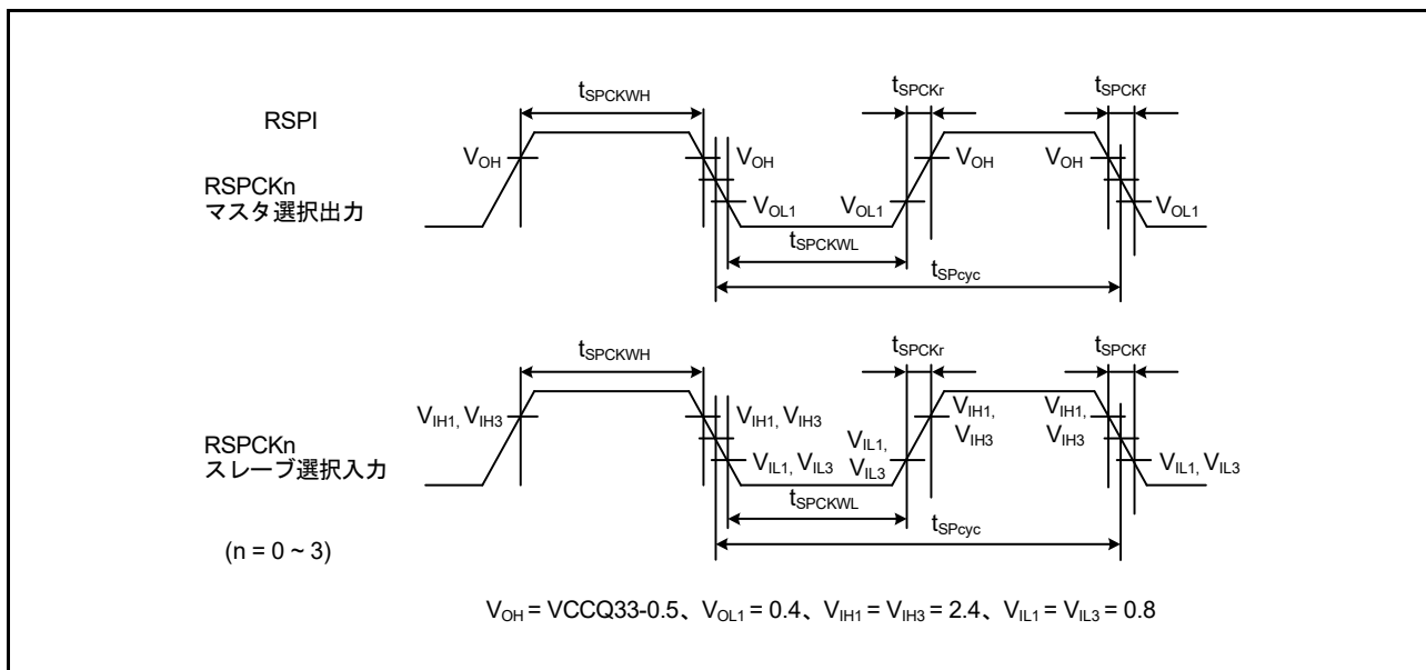
図 2.52 RSPiA クロックタイミング
