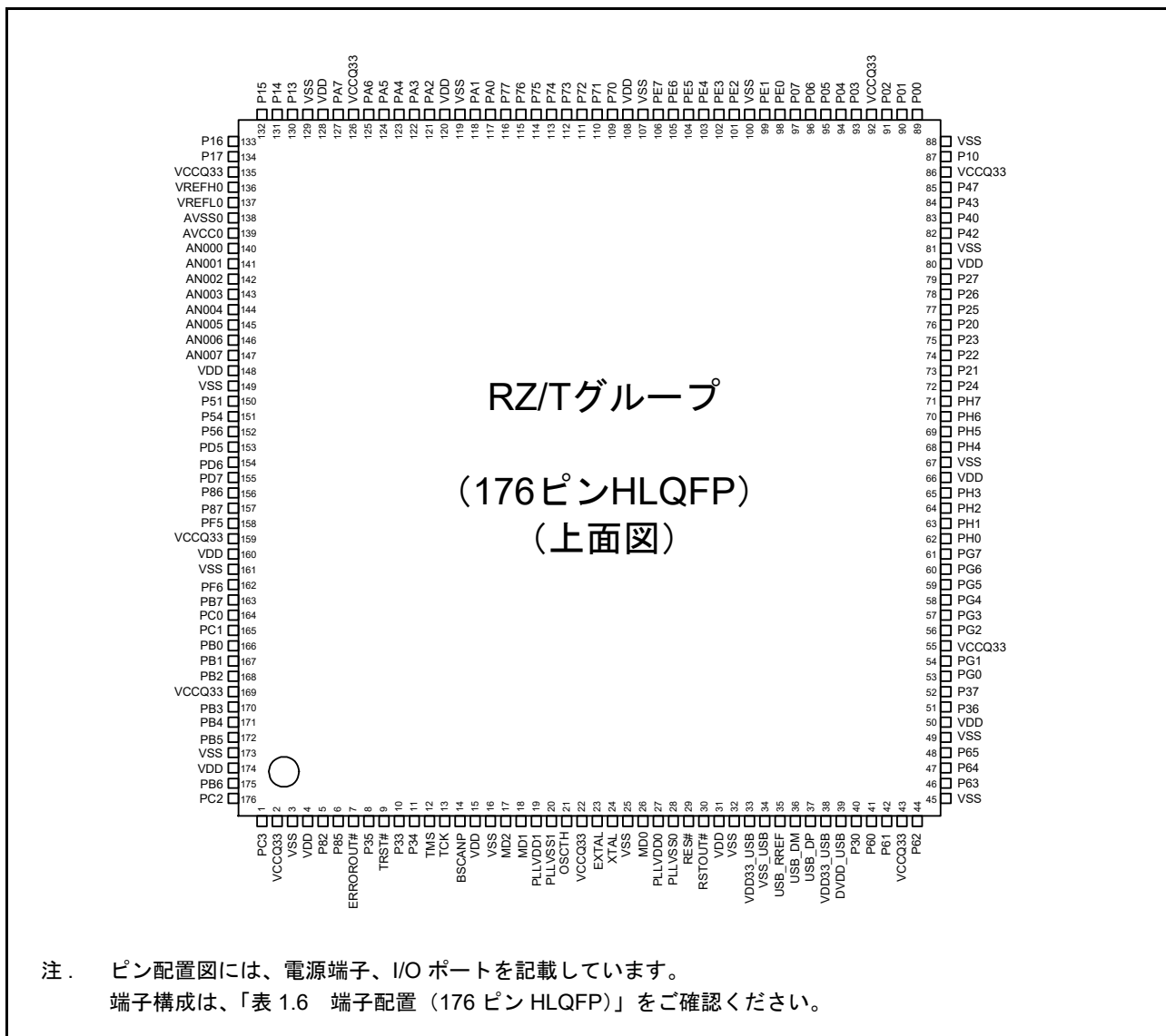
図 1.3 ピン配置図 (176 ピン HLQFP)
