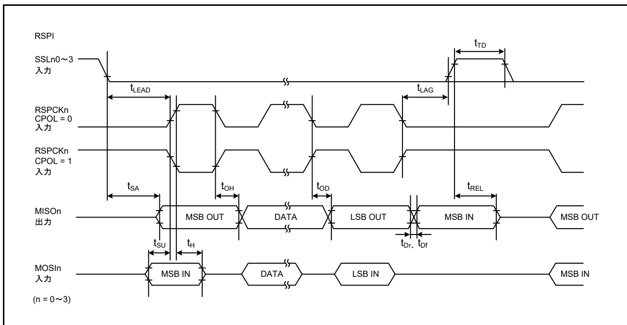
図 2.55 RSPI タイミング (スレーブ、CPHA = 0)
