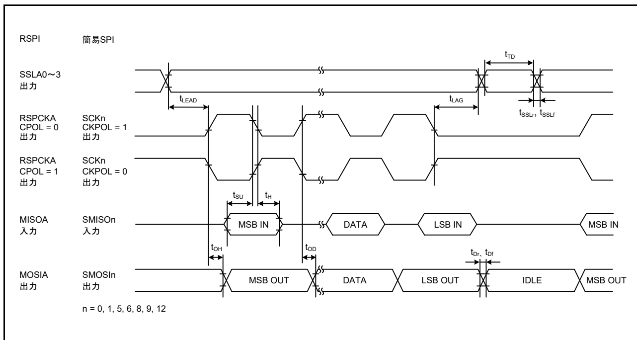
図 5.52 RSPI タイミング (マスタ、CPHA = 1)/ 簡易 SPI クロックタイミング (マスタ、CKPH = 0)
