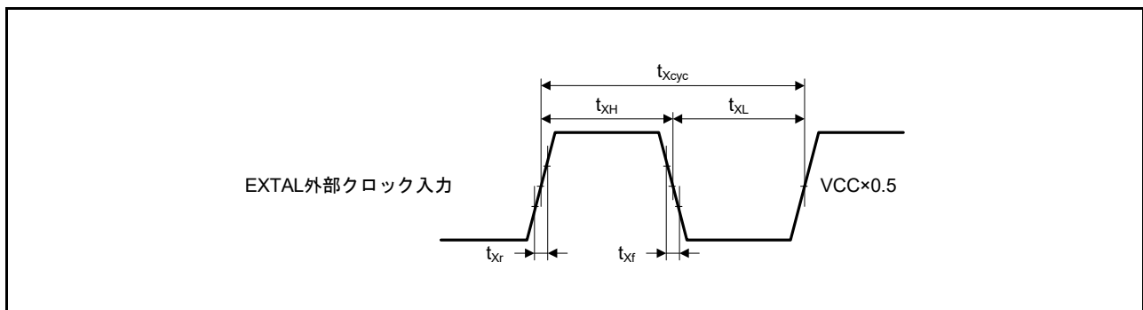
図5.26 EXTAL 外部クロック入力タイミング
