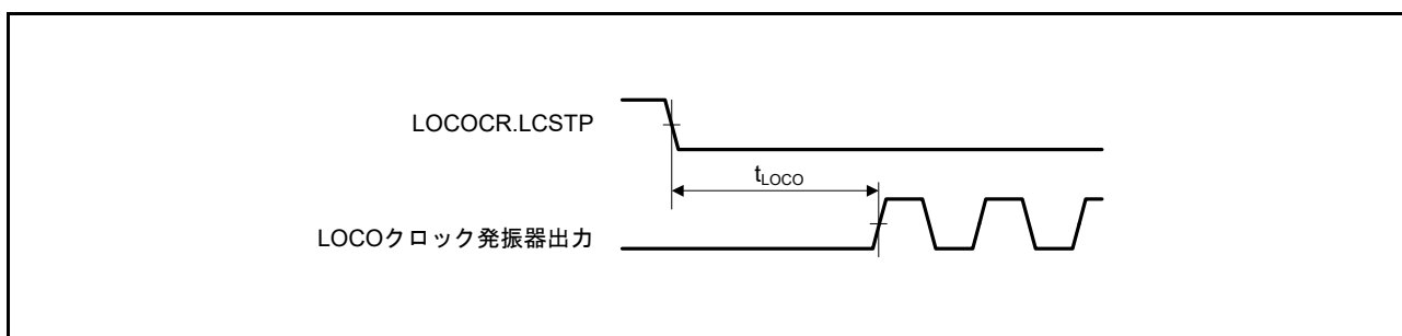
図 5.28 LOCO クロック発振開始タイミング
