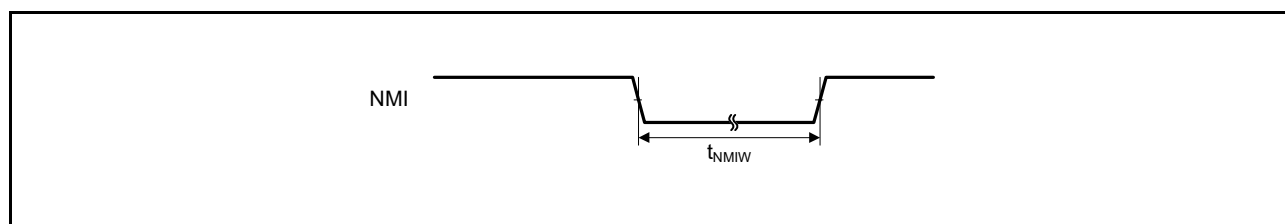
図 5.39 NMI 割り込み入力タイミング
