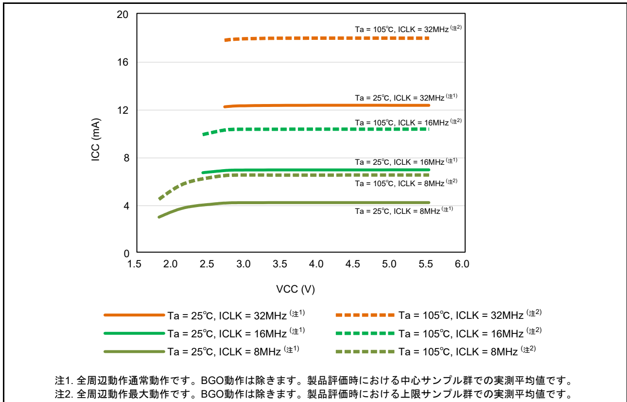
図 5.4 高速動作モードの電圧依存性 (参考データ)
