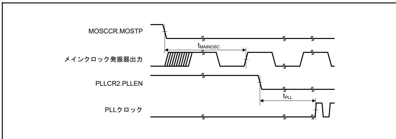
図 5.32 PLL クロック発振開始タイミング (メインクロック発振安定後に PLL を動作させたとき)
