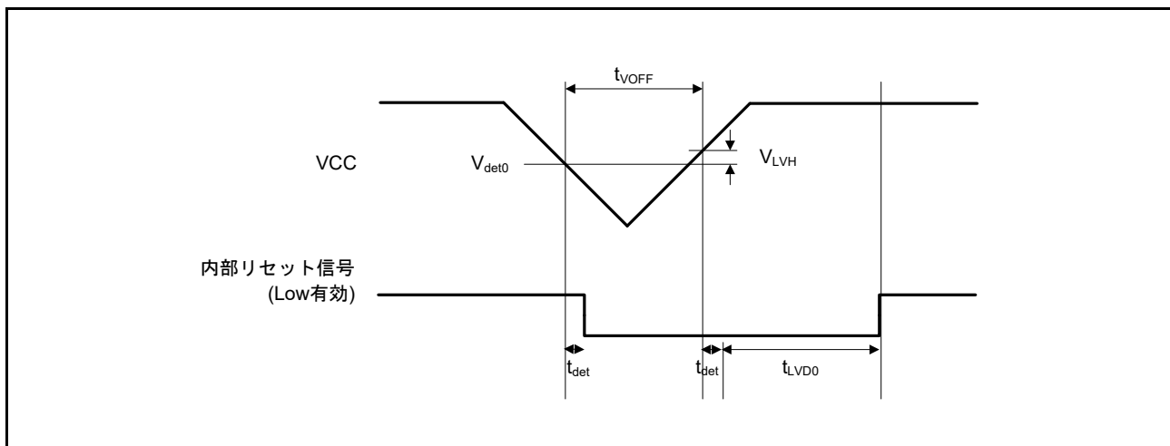
図 5.63 電圧検出回路タイミング ( V_{det0} )
