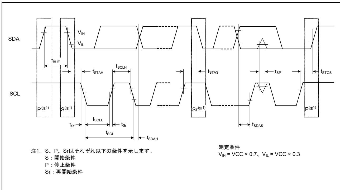
図 5.55 RIIC バスインタフェース入出力タイミング / 簡易 I 2 C バスインタフェース入出力タイミング
