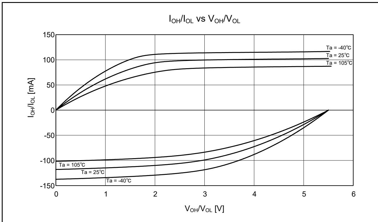
図 5.21 高駆動出力を選択したときの V_{OH}/V_{OL} 、 I_{OH}/I_{OL} 温度特性 V_{CC} = 5.5V (参考データ)
