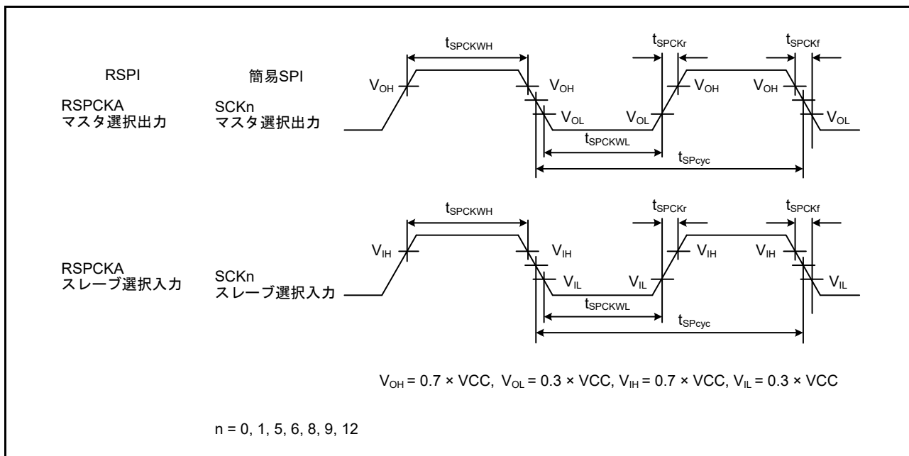
図 5.50 RSPI クロックタイミング / 簡易 SPI クロックタイミング
