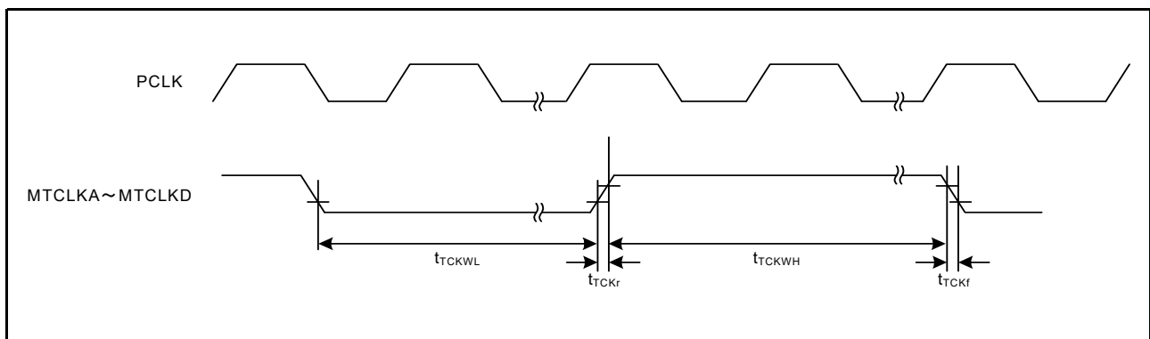
図 5.43 MTU2 クロック入力タイミング
