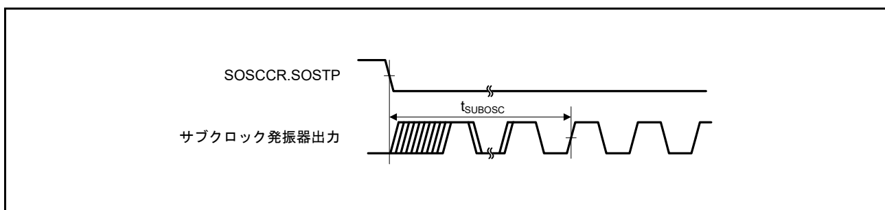
図 5.33 サブクロック発振開始タイミング
