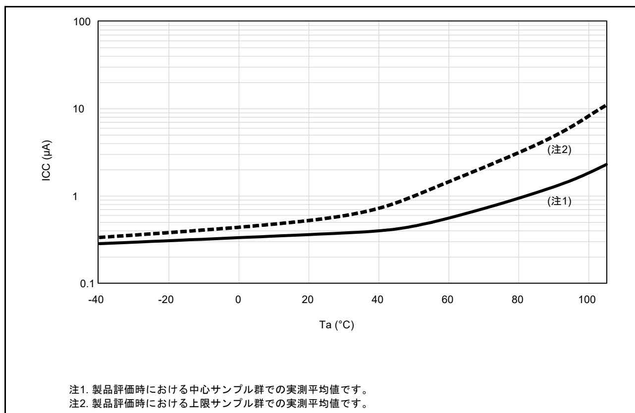
図 5.8 ソフトウェアスタンバイモード時の温度依存性 (参考データ)
