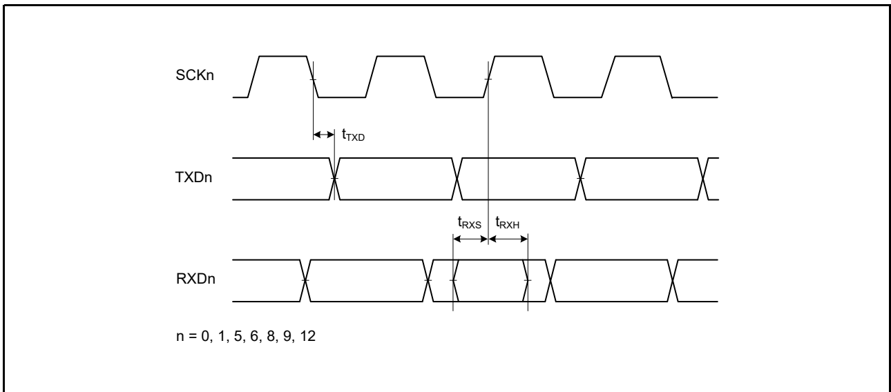
図 5.47 SCI 入出カタイミング / クロック同期式モード
