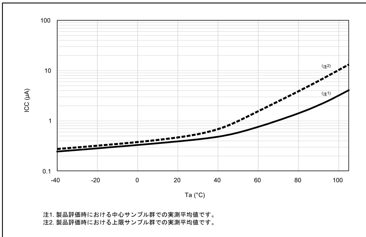
図 5.10 ソフトウェアスタンバイモード時の温度依存性 (参考データ)
