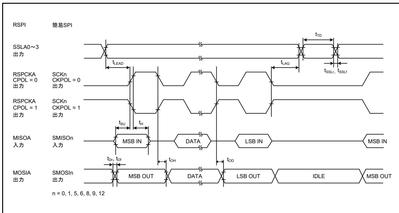
図 5.51 RSPI タイミング (マスタ、CPHA = 0)/ 簡易 SPI クロックタイミング (マスタ、CKPH = 1)
