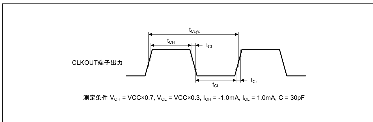
図 5.49 CLKOUT 出力タイミング
