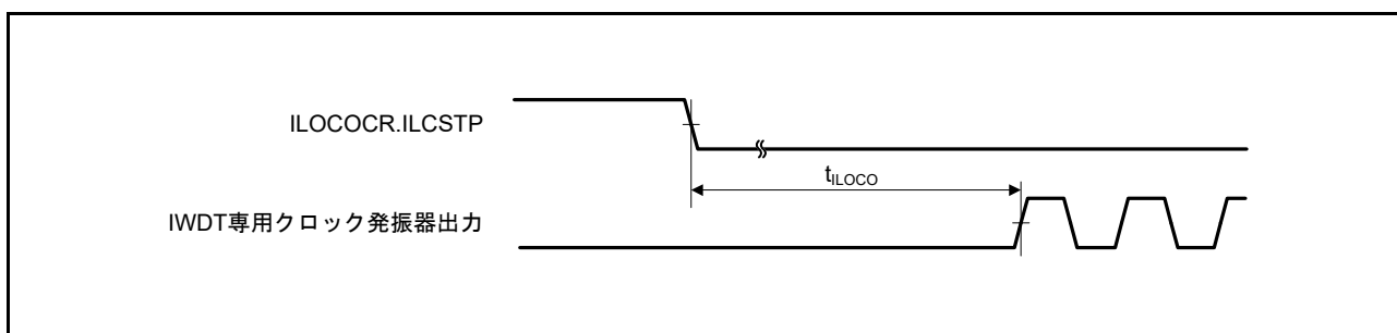
図 5.29 IWDW 専用クロック発振開始タイミング
