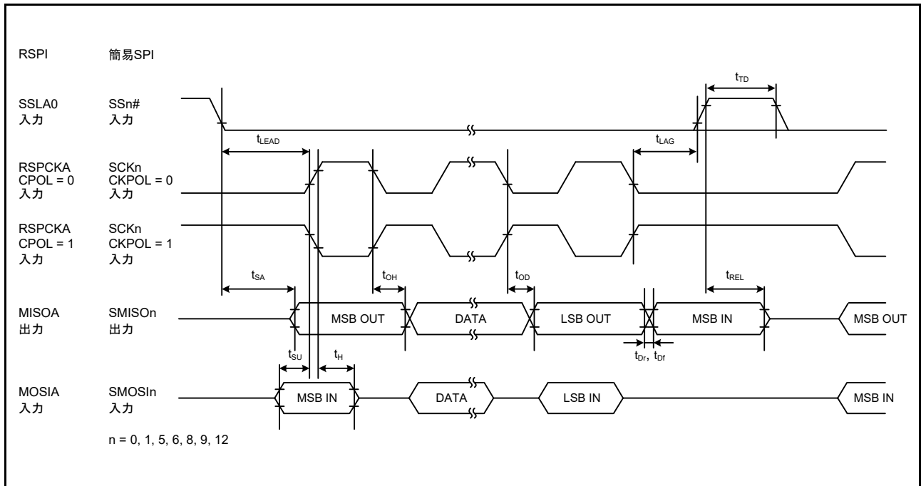
図 5.53 RSPI タイミング (スレーブ、CPHA = 0)/ 簡易 SPI クロックタイミング (スレーブ、CKPH = 1)
