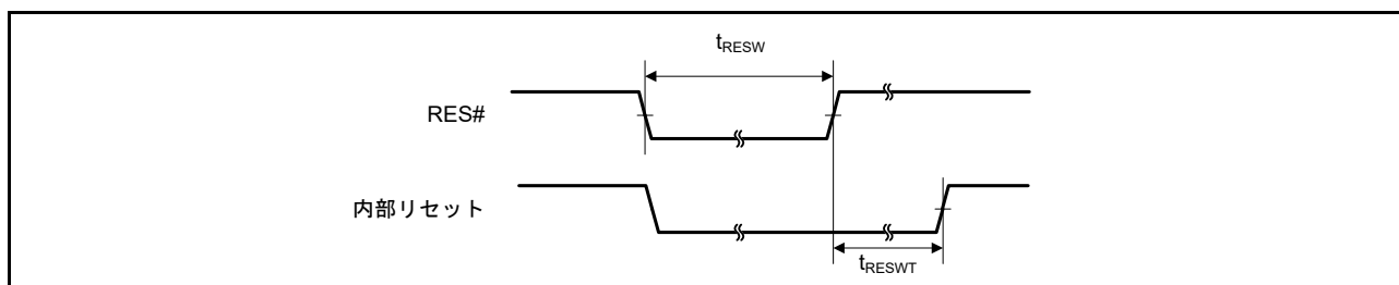
図 5.35 リセット入力タイミング (1)
