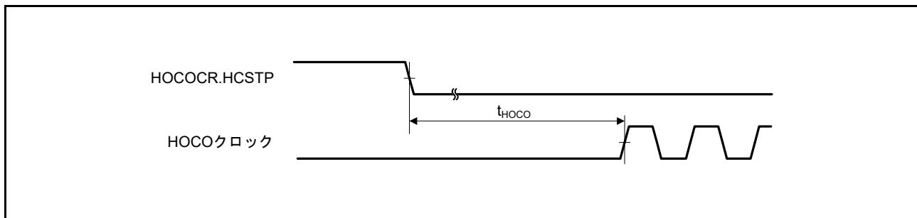
図 5.31 HOCO クロック発振開始タイミング (HOCOCR.HCSTP ビット設定による発振開始)
