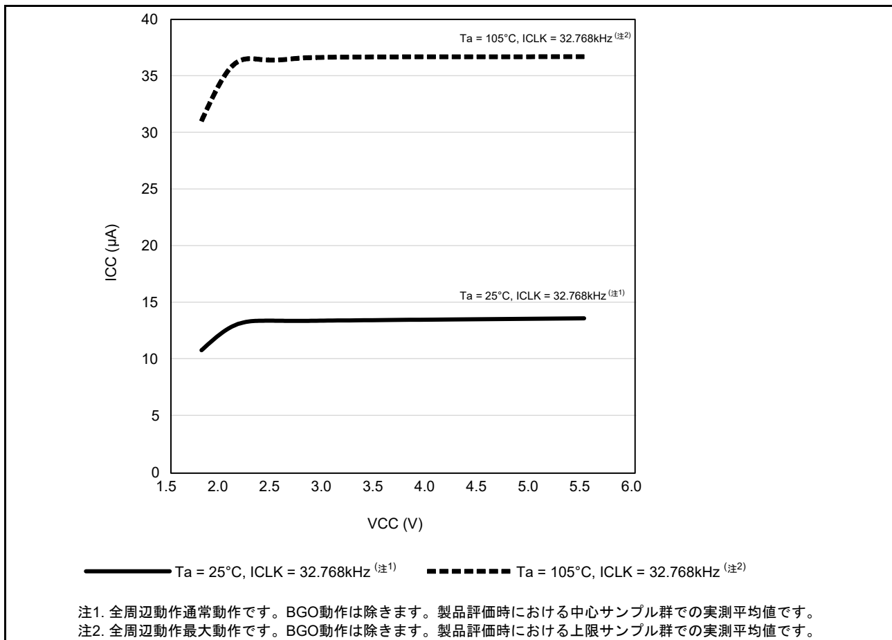
図 5.6 低速動作モードの電圧依存性 (参考データ)
