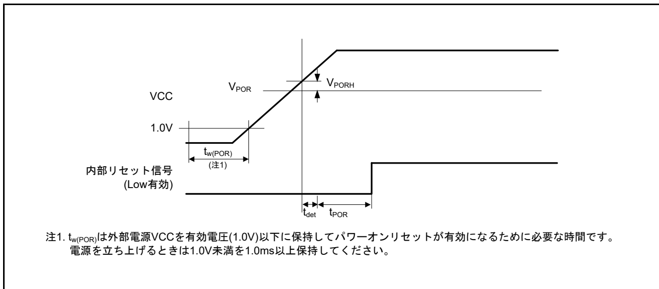
図 5.62 パワーオンリセットタイミング
