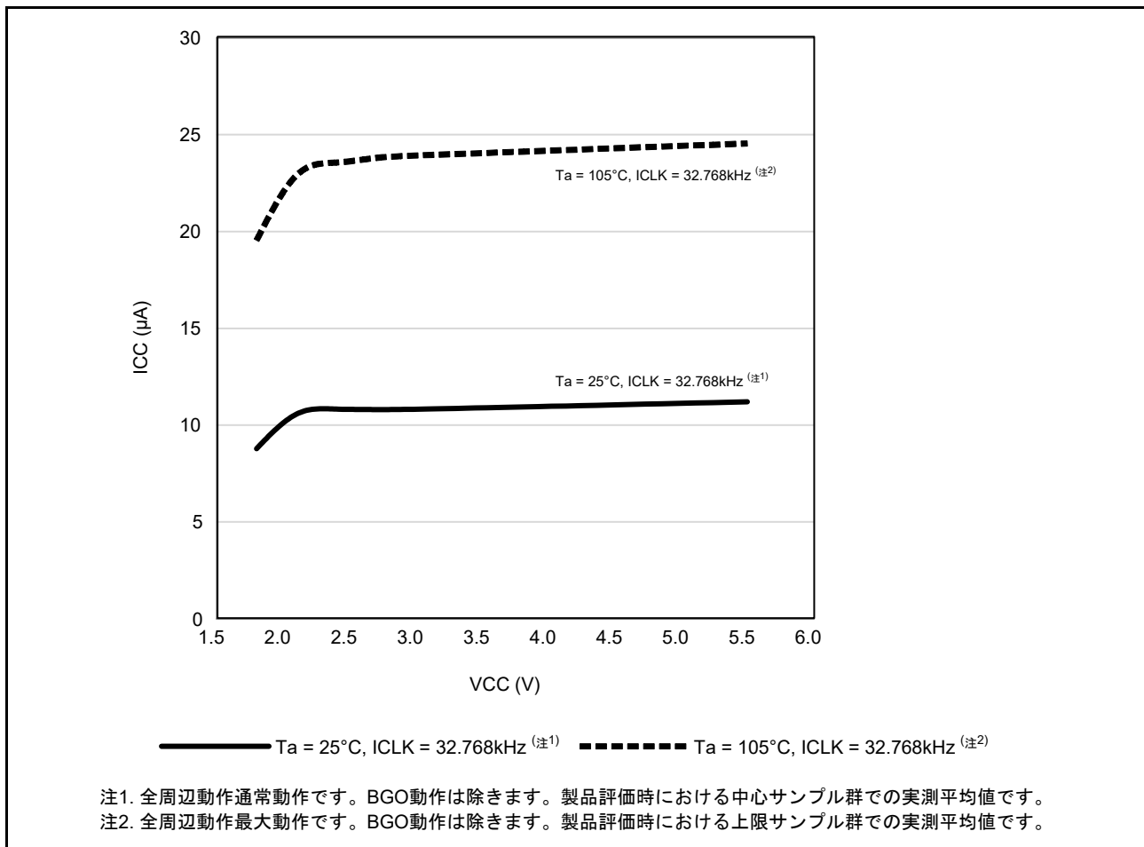
図 5.3 低速動作モードの電圧依存性 (参考データ)
