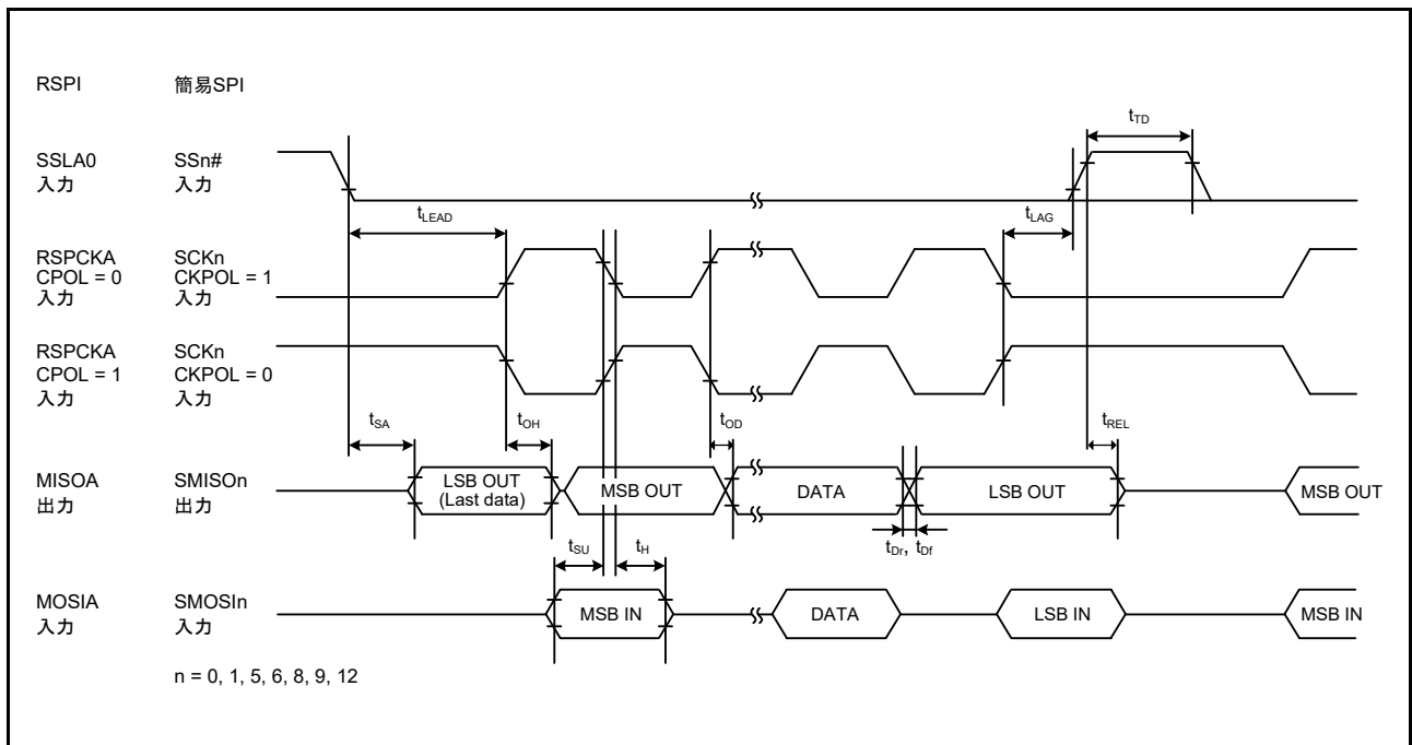
図 5.54 RSPI タイミング (スレーブ、CPHA = 1)/ 簡易 SPI クロックタイミング (スレーブ、CKPH = 0)
