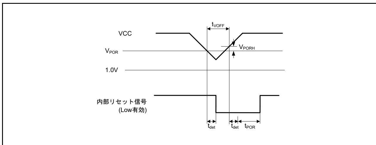
図 5.61 電圧検出リセットタイミング
