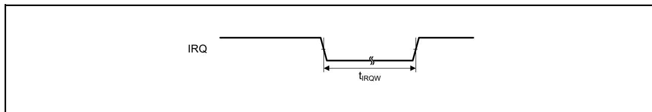
図 5.40 IRQ 割り込み入力タイミング
