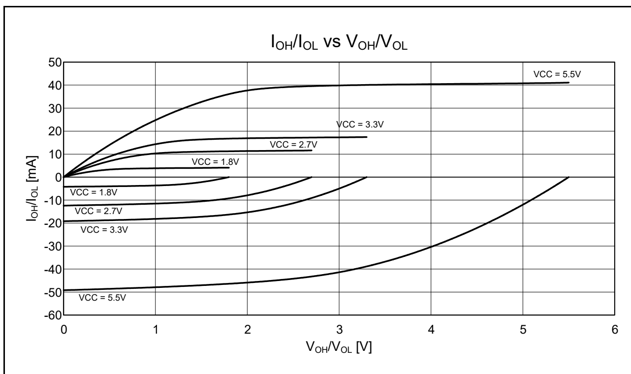
図 5.12 通常出力を選択したときの VOH/VOL、IOH/IOL 電圧特性 Ta = 25°C (参考データ)
