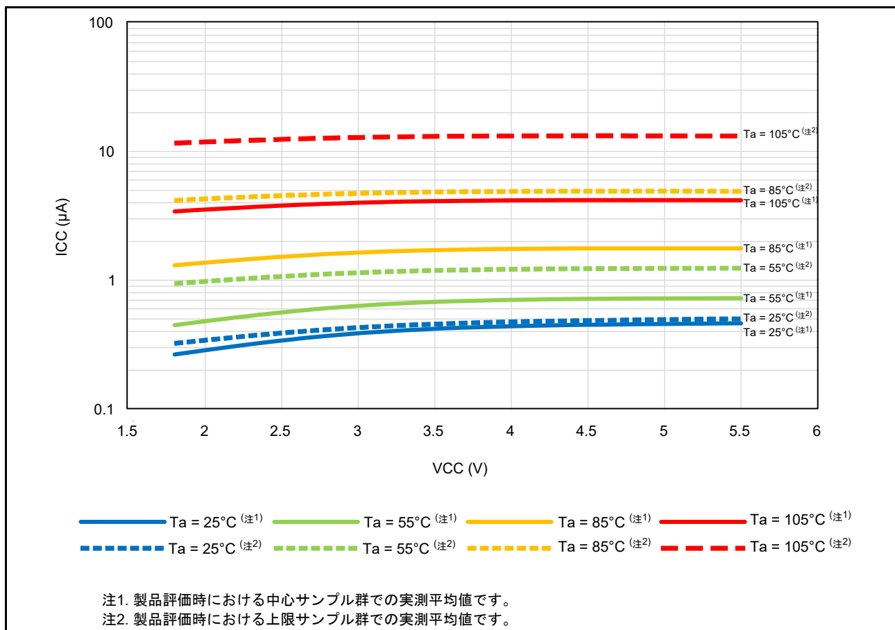
図 5.9 ソフトウェアスタンバイモード時の電圧依存性 (参考データ)
