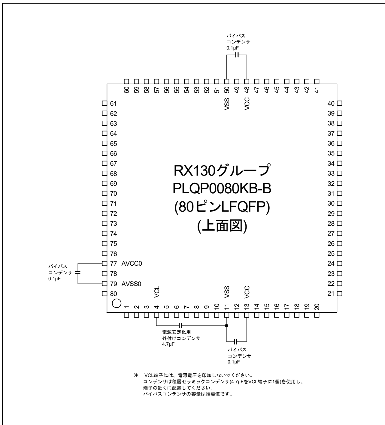
図 5.68 コンデンサ接続方法 (80ピン)
