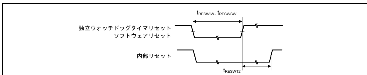
図 5.36 リセット入力タイミング (2)
