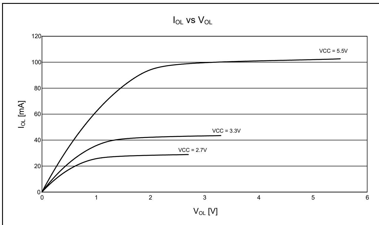
図 5.22 RIIC 出力端子の V OL 、I OL 電圧特性 T a = 25°C (参考データ)
