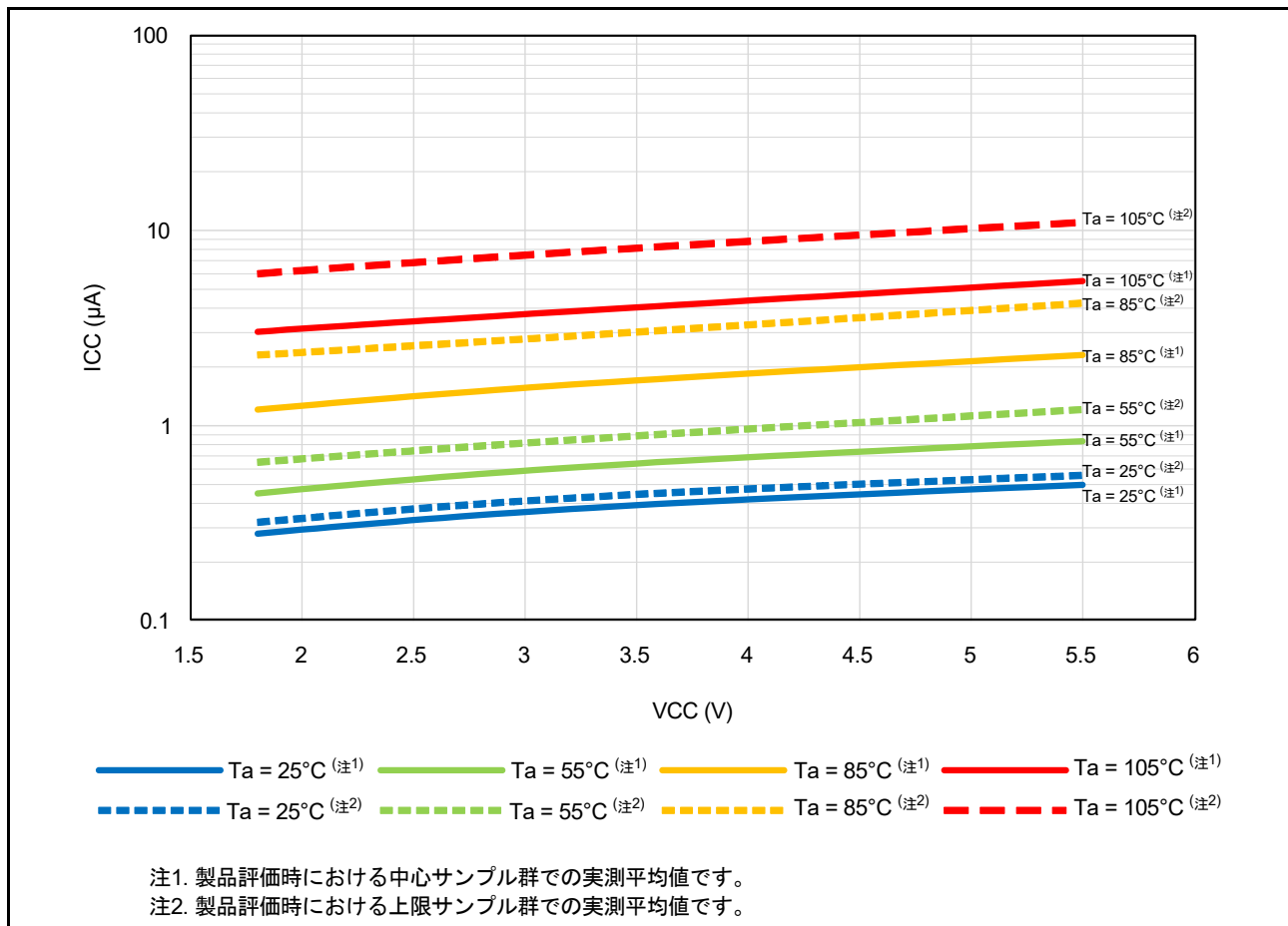
図 5.7 ソフトウェアスタンバイモード時の電圧依存性 (参考データ)
