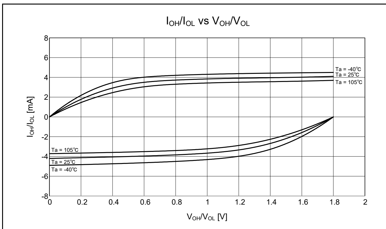
図 5.13 通常出力を選択したときの VOH/VOL、IOH/IOL 温度特性 VCC = 1.8V (参考データ)
