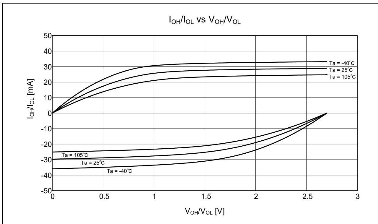
図 5.19 高駆動出力を選択したときの V_{OH}/V_{OL} 、 I_{OH}/I_{OL} 温度特性 V_{CC} = 2.7V (参考データ)
