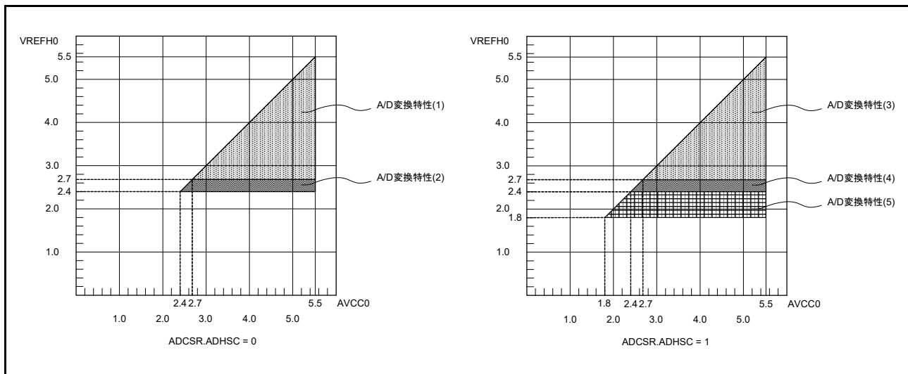
図 5.56 AVCC0-VREFH0 電圧範囲
