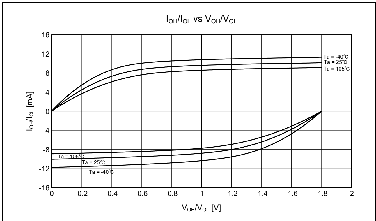
図 5.18 高駆動出力を選択したときの V_{OH}/V_{OL} 、 I_{OH}/I_{OL} 温度特性 V_{CC} = 1.8\text{V} (参考データ)
