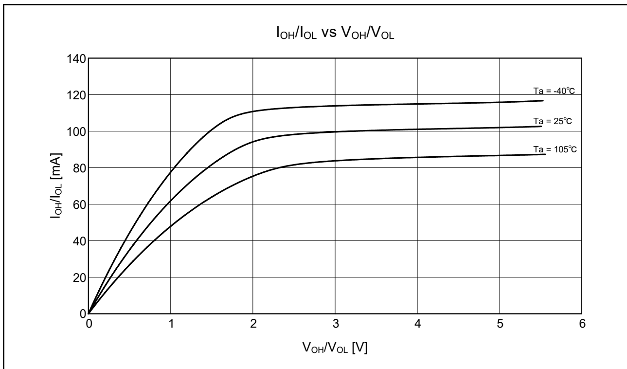
図 5.25 RIIC 出力端子の V OL 、I OL 温度特性 VCC = 5.5V (参考データ)
