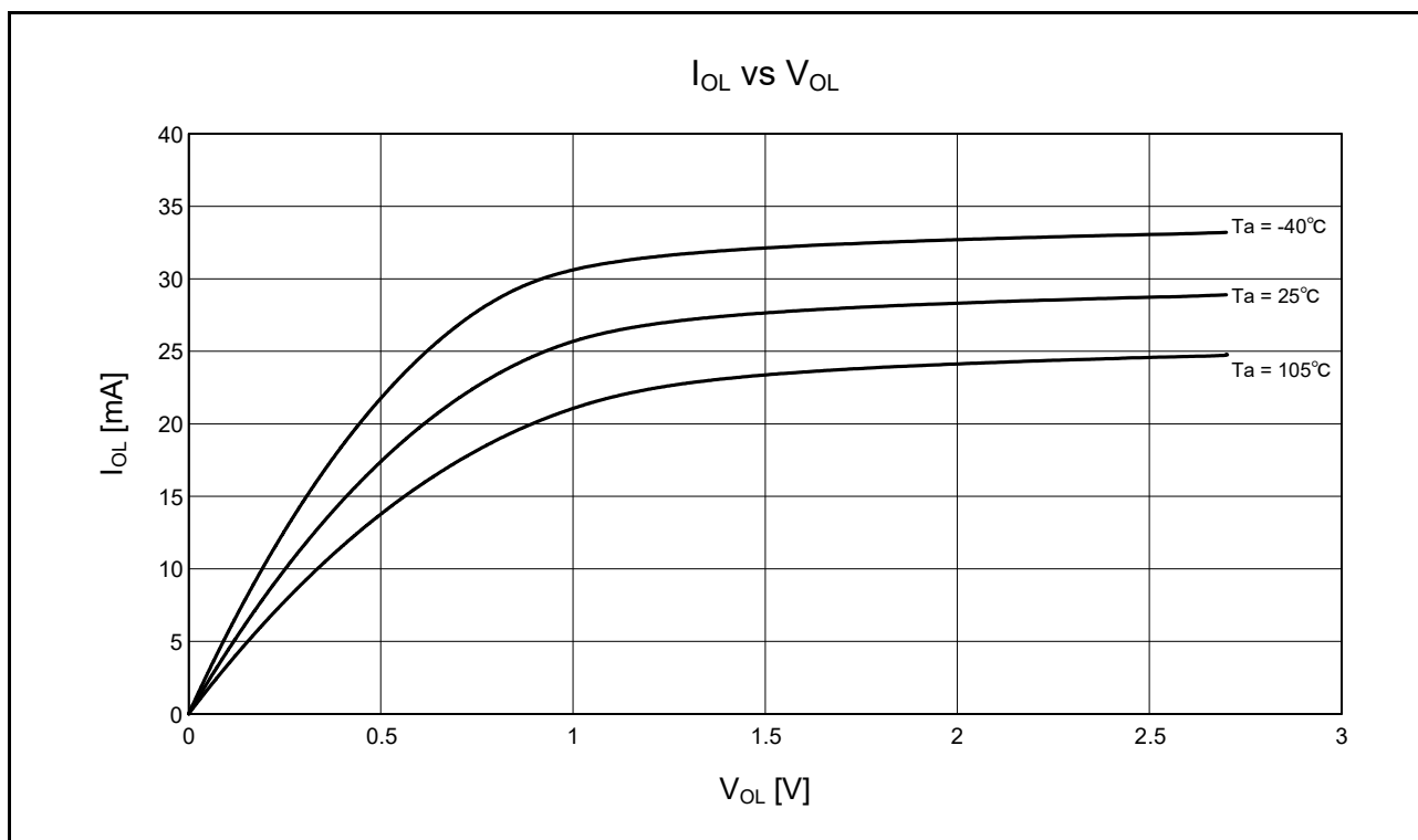
図 5.23 RIIC 出力端子の V OL 、I OL 温度特性 VCC = 2.7V (参考データ)
