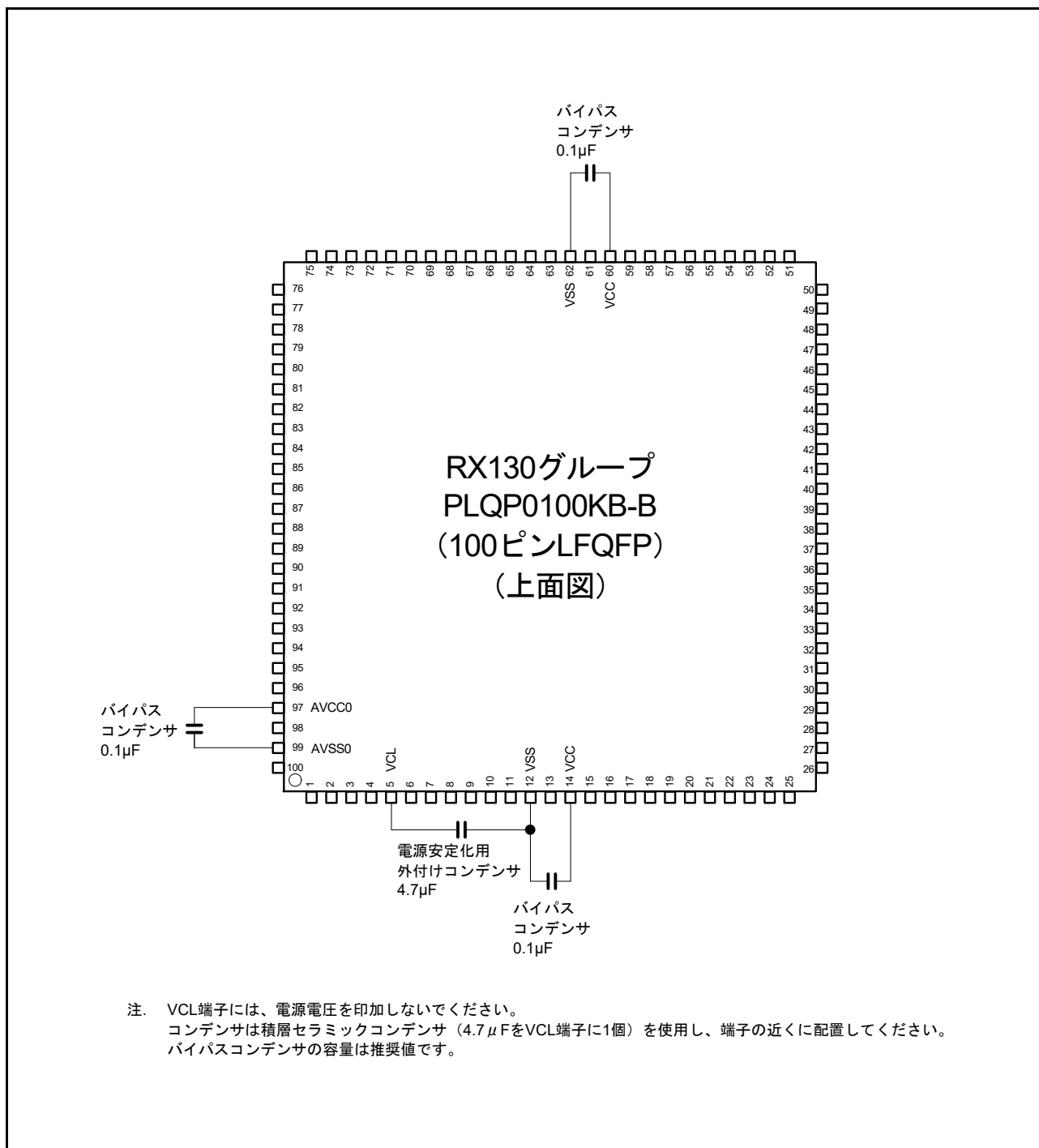
図 5.67 コンデンサ接続方法 (100 ピン)
