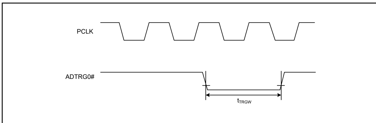
図 5.48 A/D コンバータ外部トリガ入力タイミング
