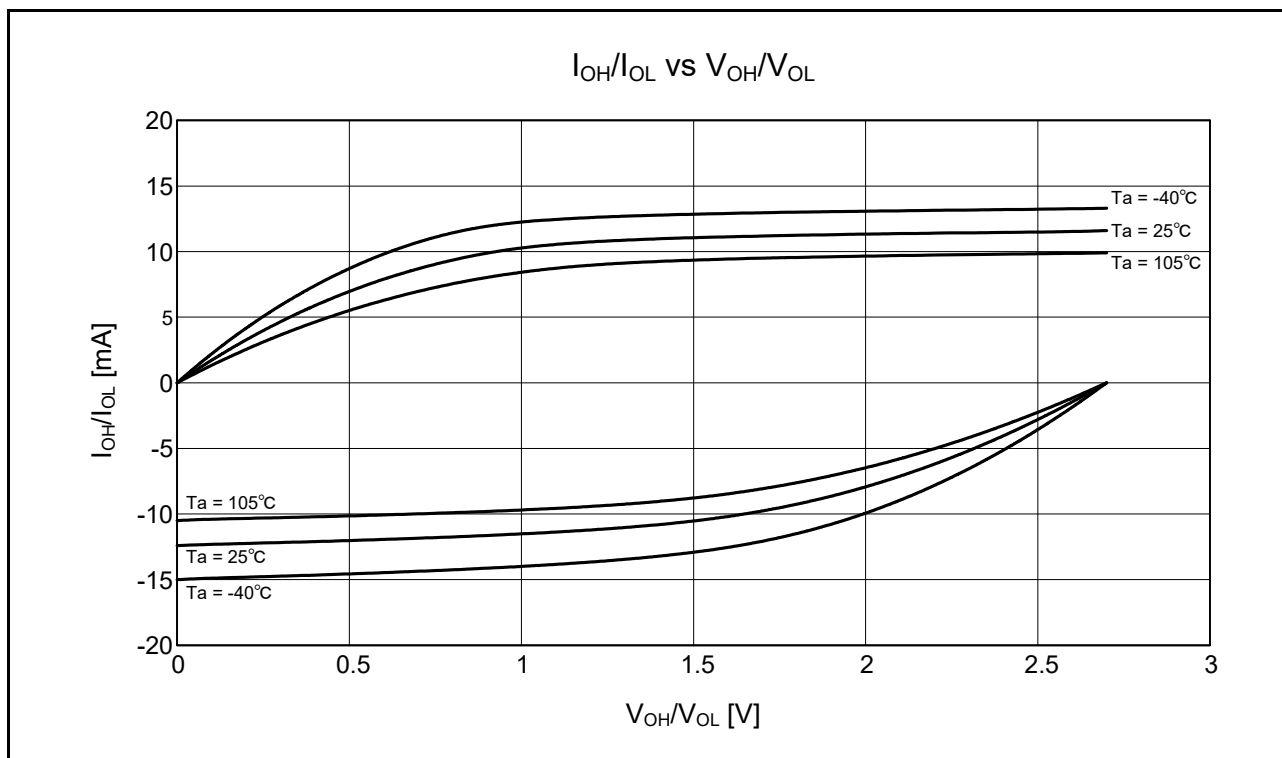
図 5.14 通常出力を選択したときの V_{OH}/V_{OL} 、 I_{OH}/I_{OL} 温度特性 V_{CC} = 2.7V (参考データ)
