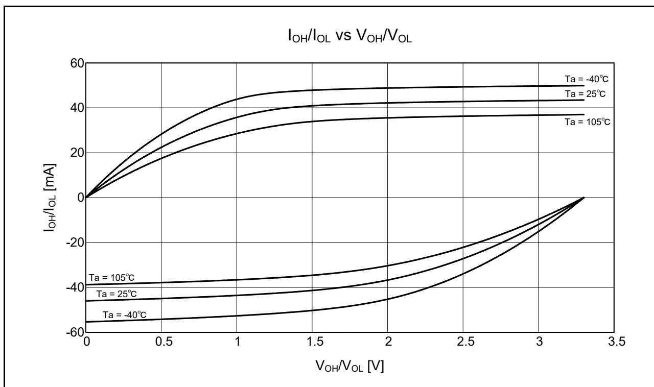
図 5.20 高駆動出力を選択したときの V_{OH}/V_{OL} 、 I_{OH}/I_{OL} 温度特性 V_{CC} = 3.3V (参考データ)
