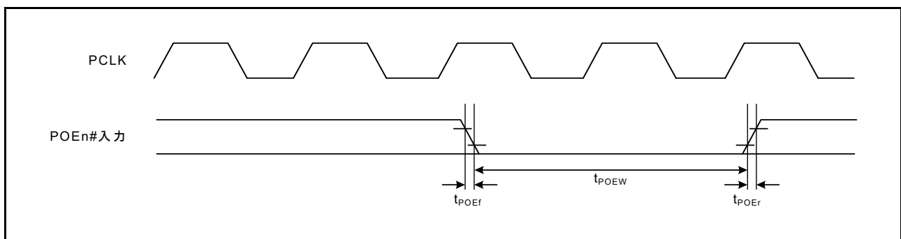
図 5.44 POE# 入力タイミング
