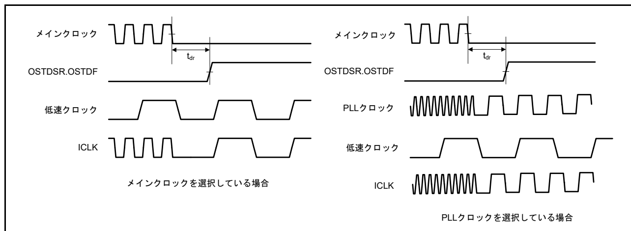
図 5.66 発振停止検出タイミング
