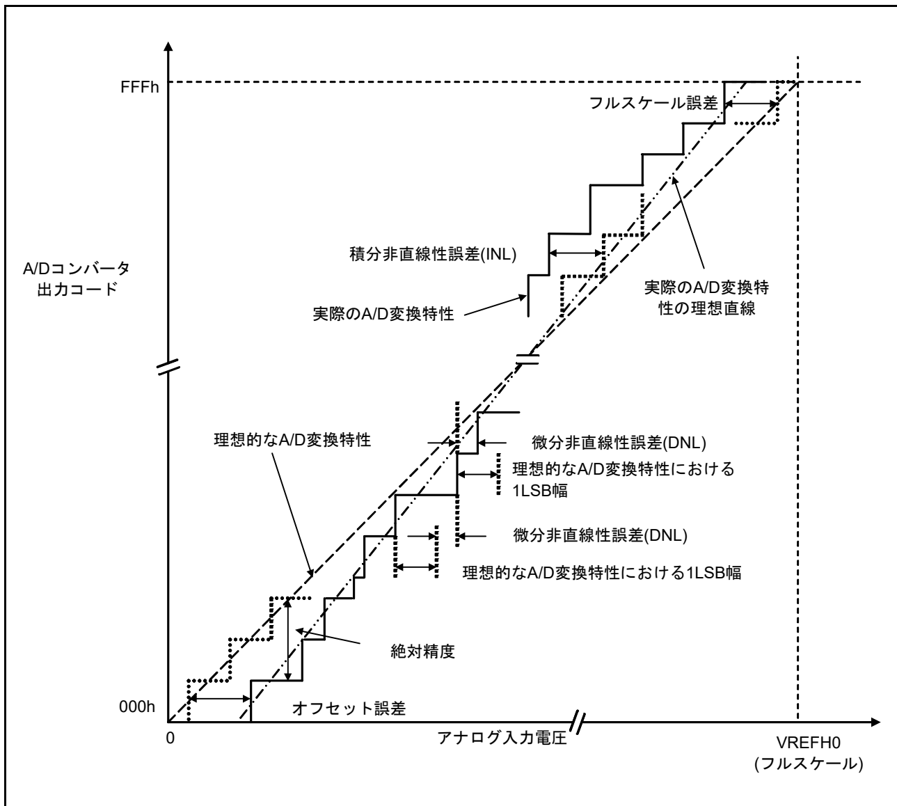
図 5.58 A/D コンバータ特性用語説明図
