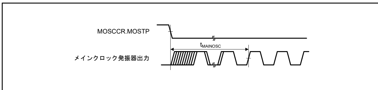
図 5.27 メインクロック発振開始タイミング
