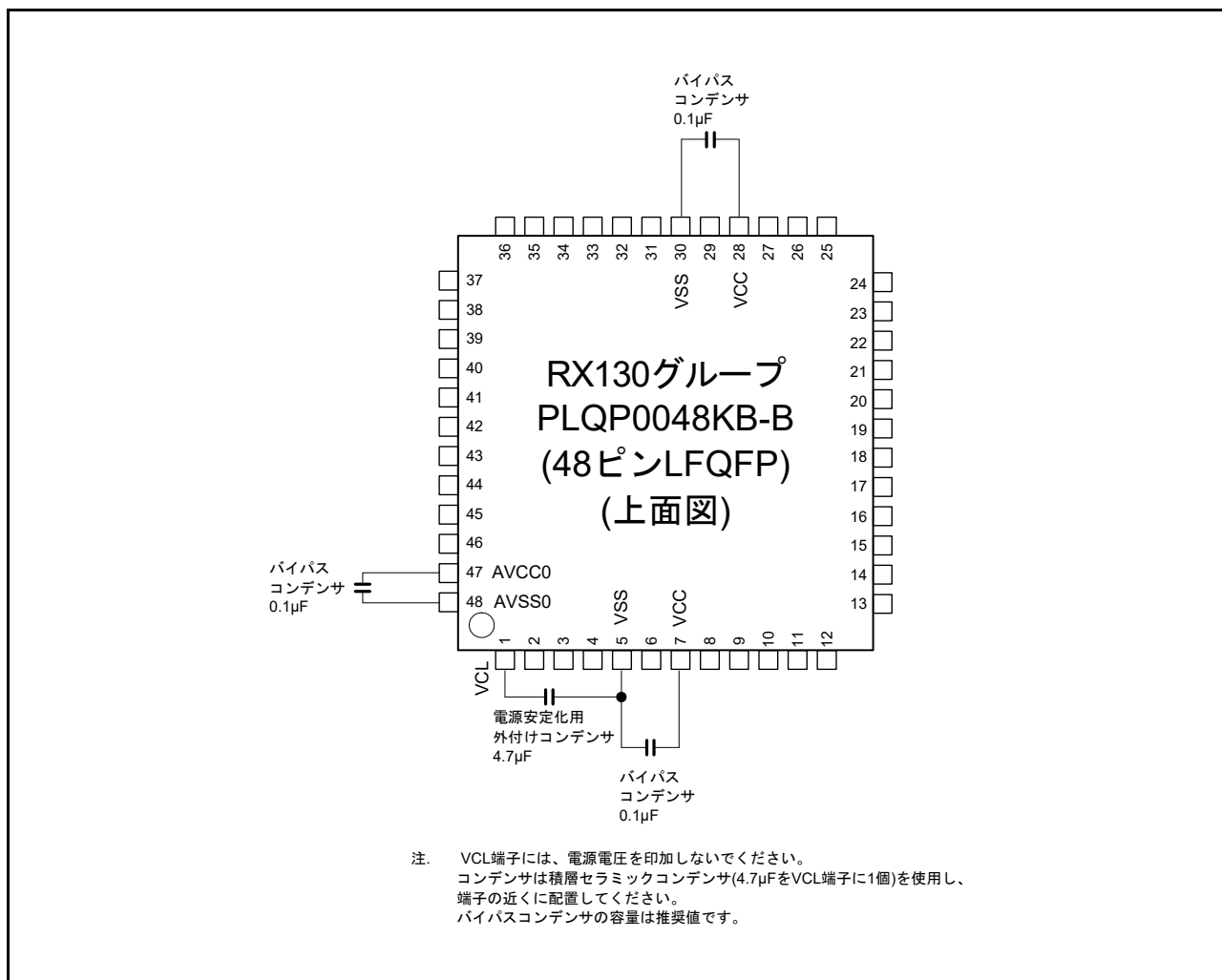
図 5.70 コンデンサ接続方法 (48 ピン)
