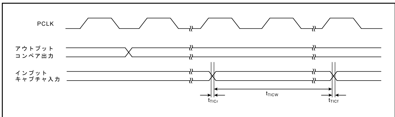
図 5.42 MTU2 入出力タイミング
