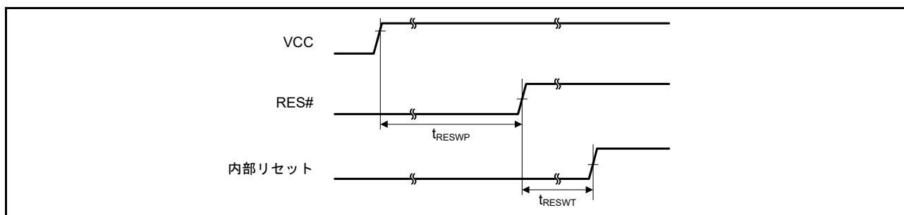
図 5.34 電源投入時リセット入力タイミング
