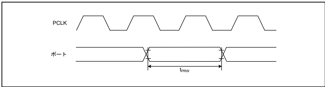
図 5.41 I/O ポート入力タイミング
