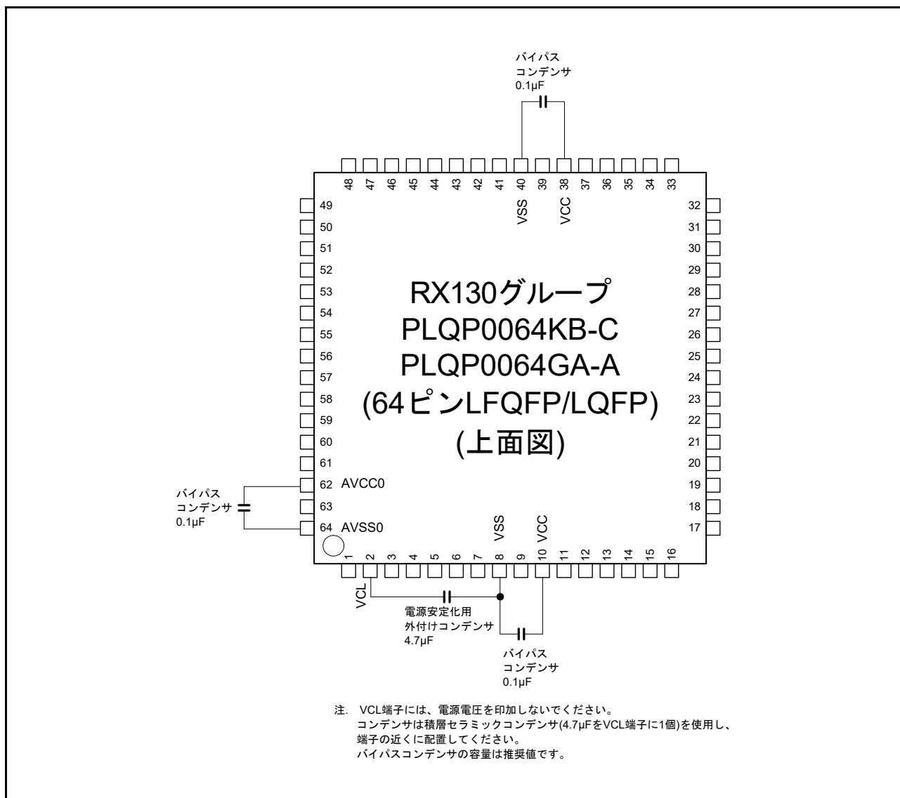
図 5.69 コンデンサ接続方法 (64 ピン)
