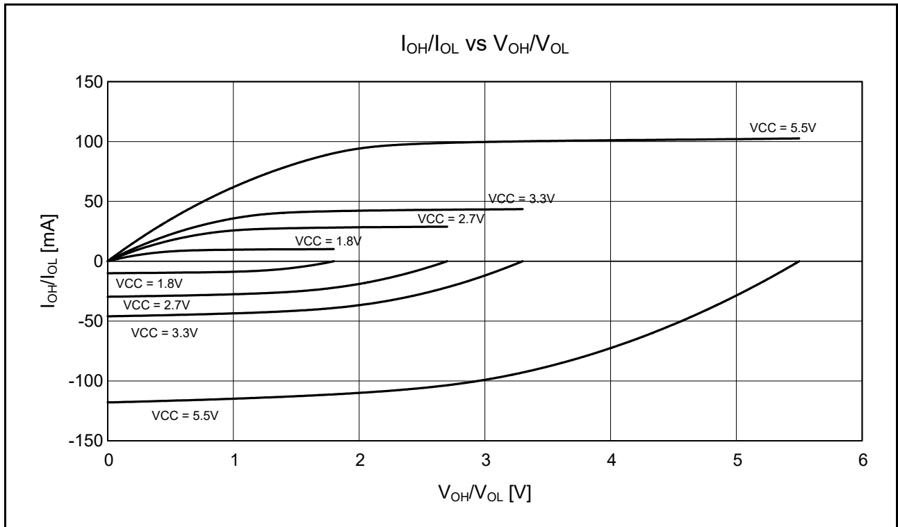
図 5.17 高駆動出力を選択したときの V_{OH}/V_{OL} 、 I_{OH}/I_{OL} 電圧特性 T_a = 25^\circ\text{C} (参考データ)
