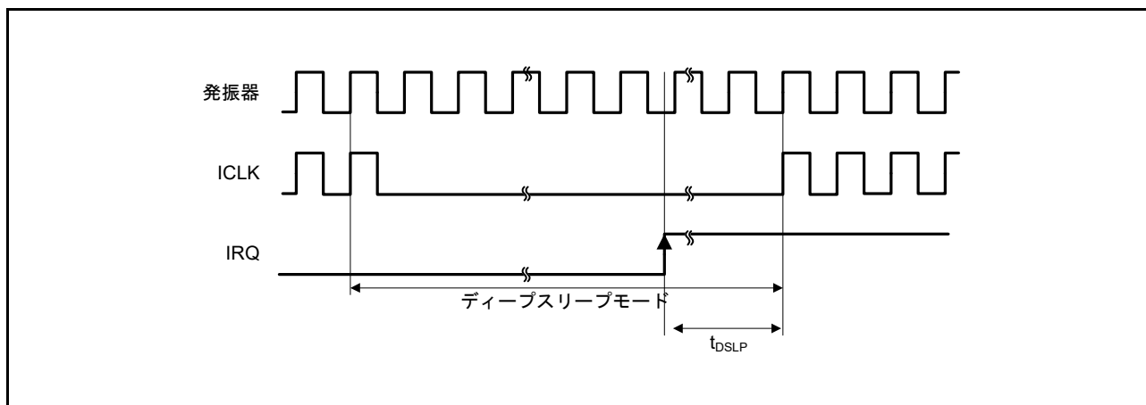
図 5.38 ディープスリープモード解除タイミング
