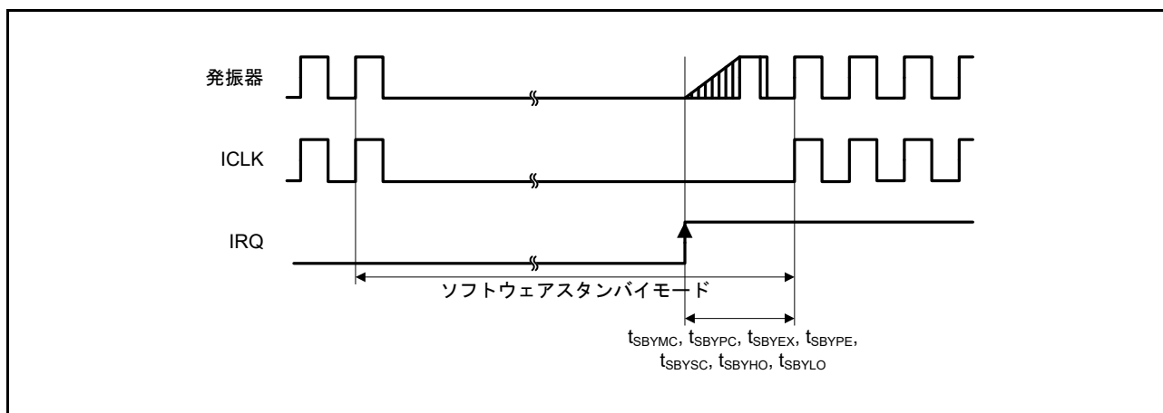
図 5.37 ソフトウェアスタンバイモード復帰タイミング
