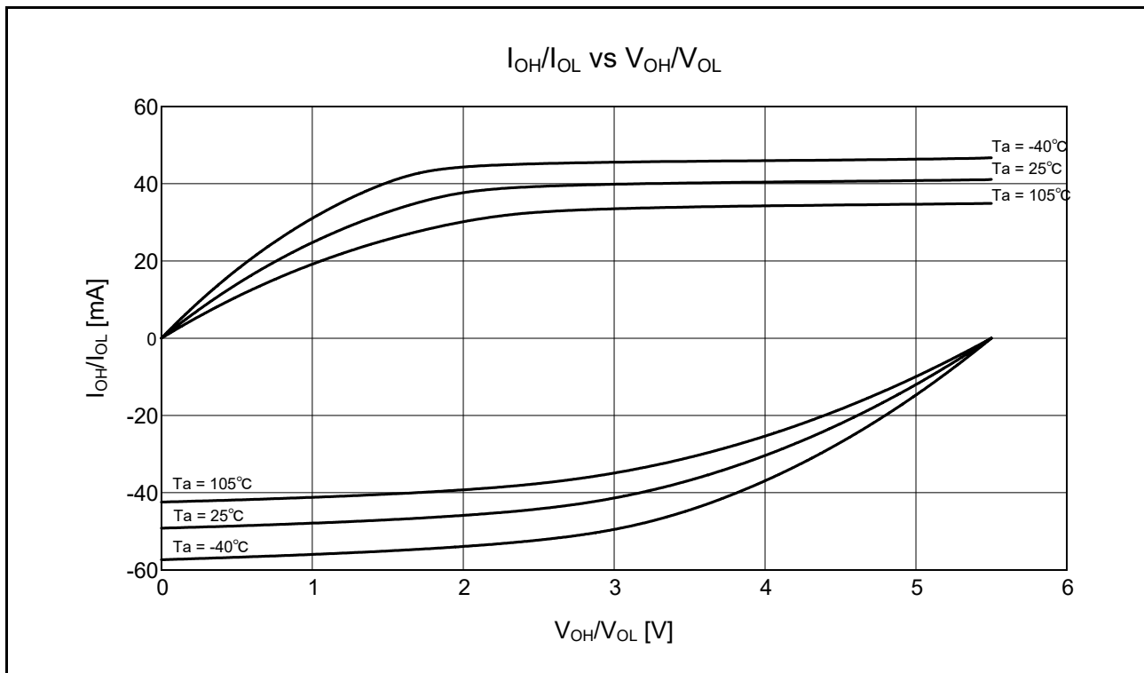
図 5.16 通常出力を選択したときの V OH /V OL 、I OH /I OL 温度特性 VCC = 5.5V (参考データ)
