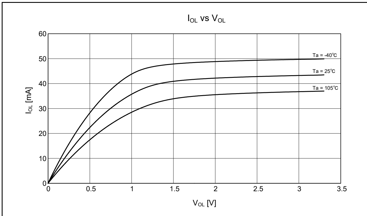
図 5.24 RIIC 出力端子の V OL 、I OL 温度特性 VCC = 3.3V (参考データ)
