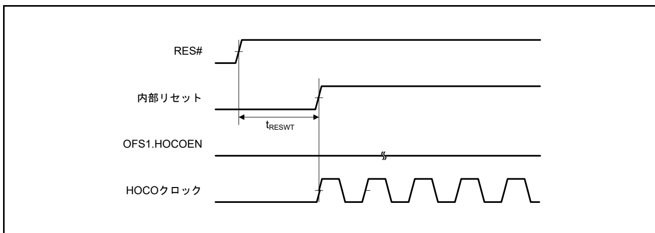
図 5.30 HOCO クロック発振開始タイミング (OFS1.HOCOEN ビット “0” 設定時のリセット解除後)
