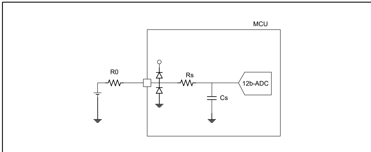
図 5.57 等価回路
