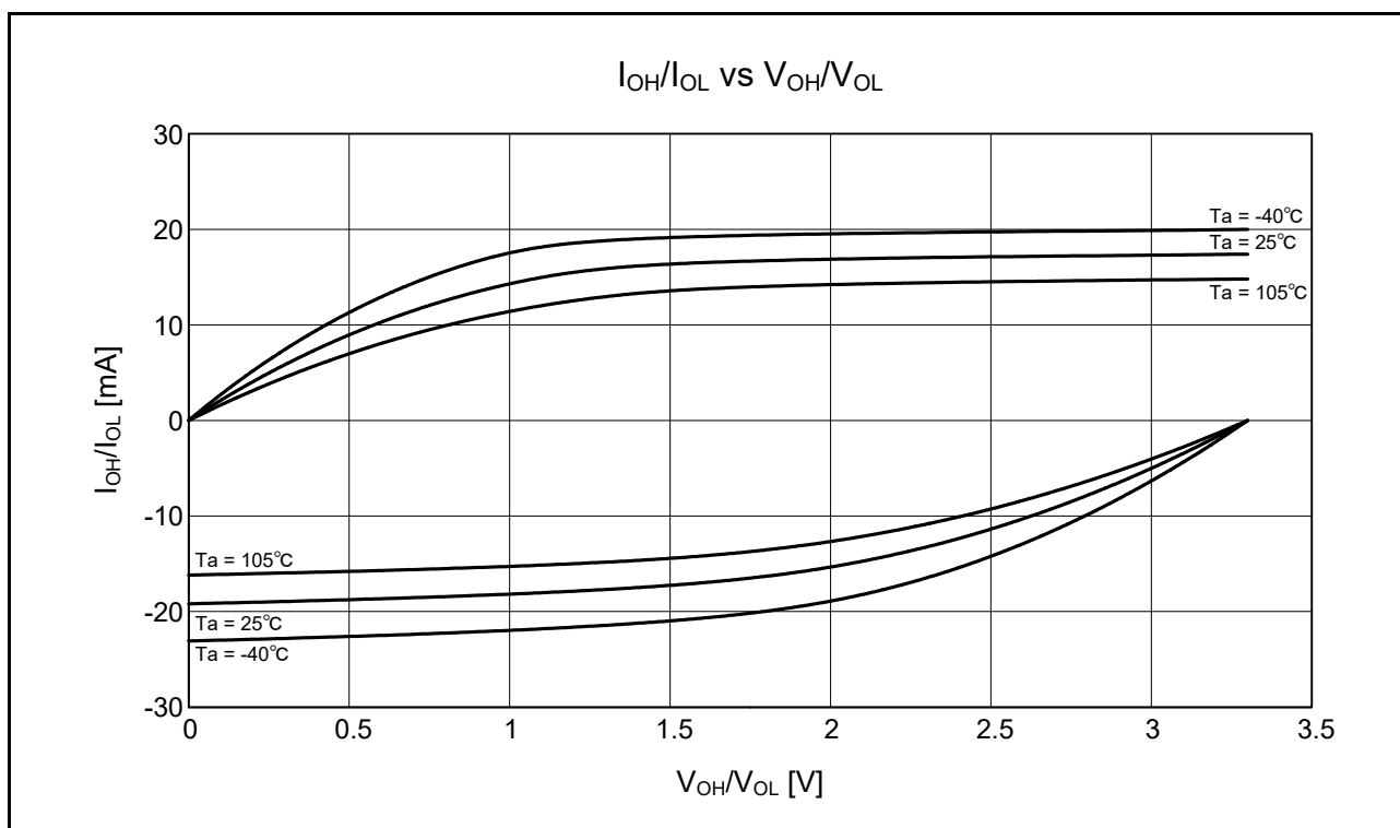
図 5.15 通常出力を選択したときの V_{OH}/V_{OL} 、 I_{OH}/I_{OL} 温度特性 V_{CC} = 3.3V (参考データ)
