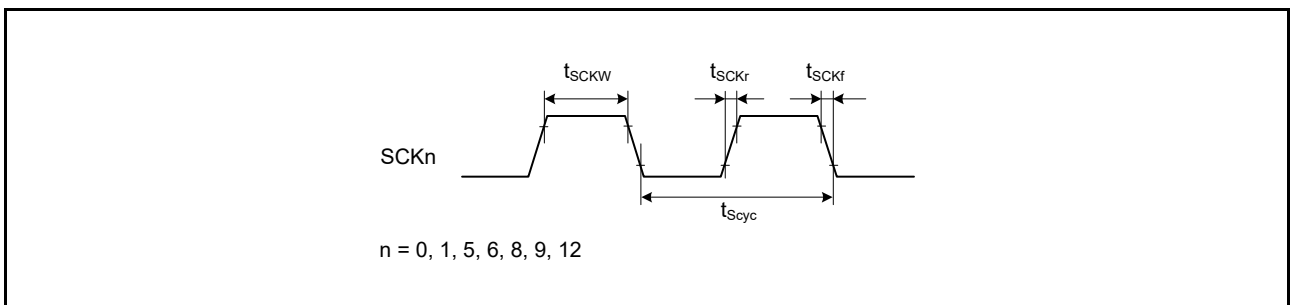
図 5.46 SCK クロック入カタイミング
