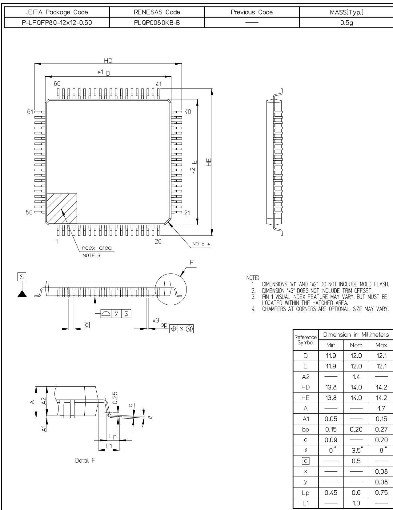
図 B. 80 ピン LFQFP (PLQP0080KB-B)
