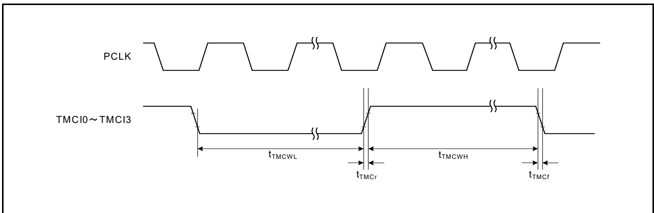
図 5.45 TMR クロック入カタイミング
