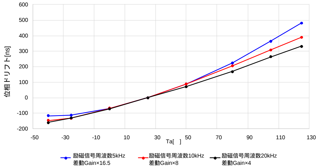
図 6.1 位相ドリフト (vs 温度)
