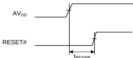
図 5.3 リセット入力タイミング (1)
