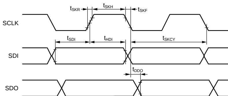
図 5.6 SPI タイミング
