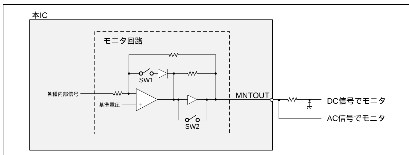
図 2.7 モニタ端子外付け回路構成例
