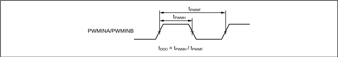
図 5.7 位相調整信号入力タイミング
