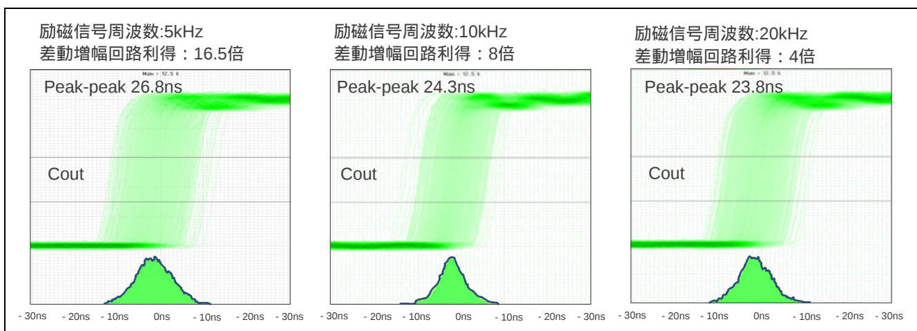
図 6.2 出力ジッタ幅 (ヒストグラム)
