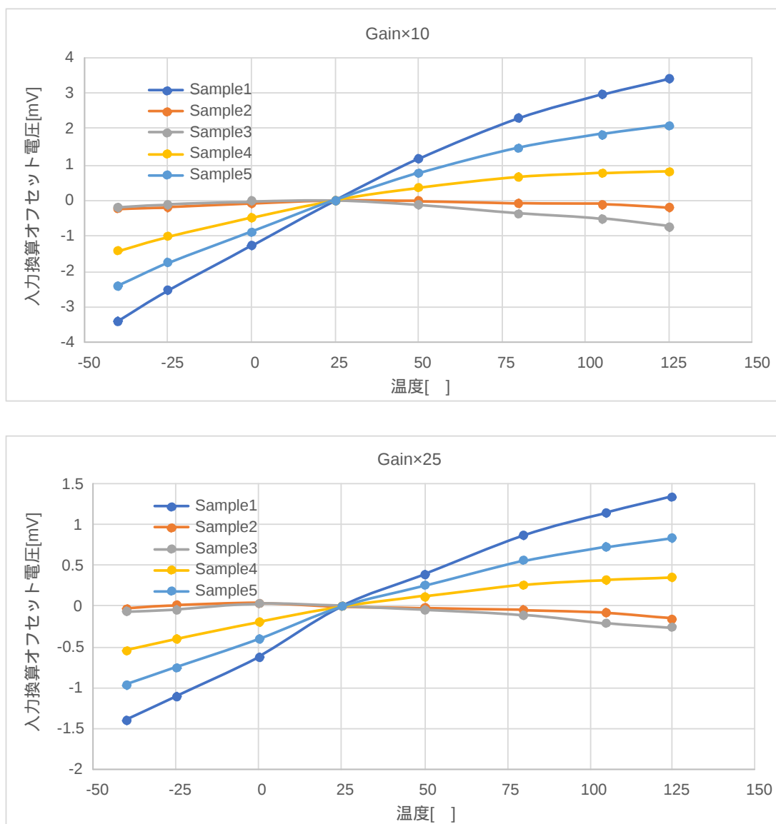
図 6.3 シャント電流増幅回路オペアンプオフセットドリフト (vs 温度) (1/2)
