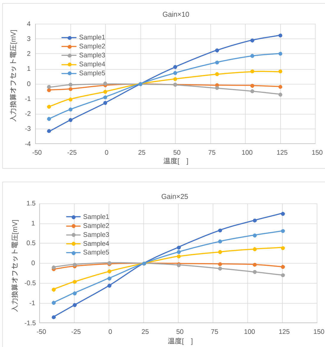
図 6.3 シャント電流増幅回路オペアンプオフセットドリフト (vs 温度) (2/2)
