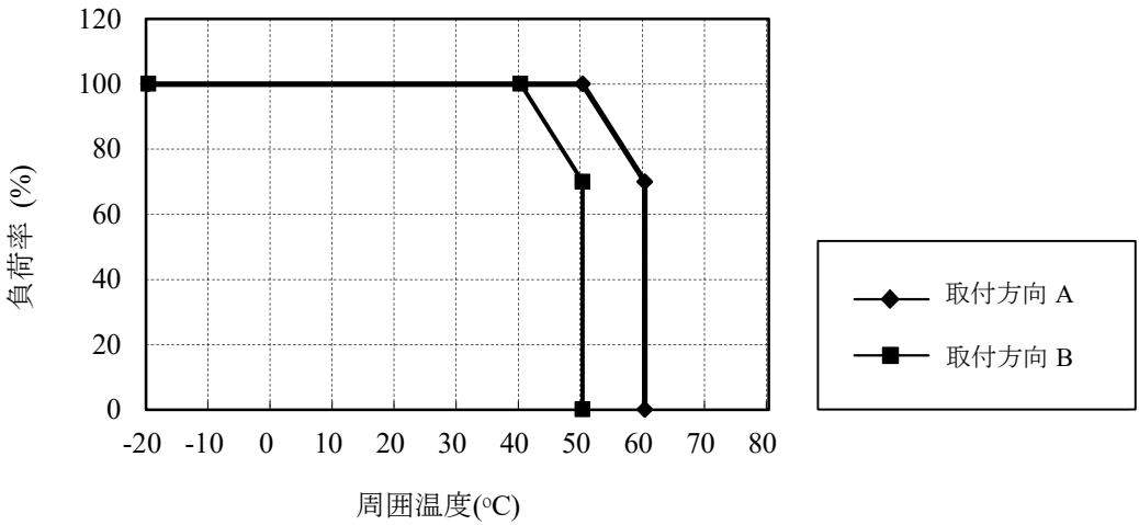
出力デレレーティングカーブ
