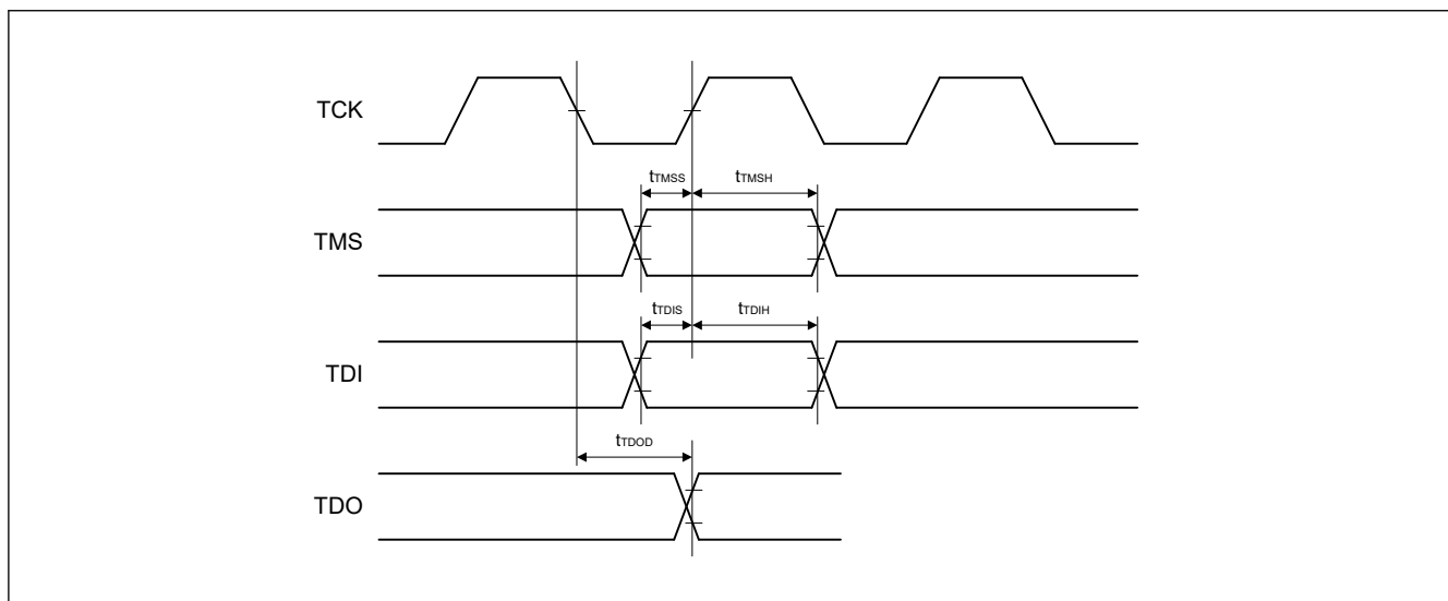
図 2.64 バウンダリスキャン入出力タイミング
