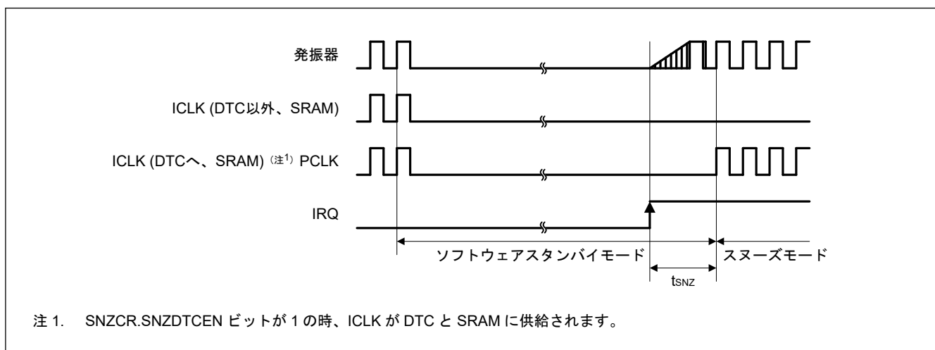
図 2.16 ソフトウェアスタンバイモードからスヌーズモードへの復帰タイミング
