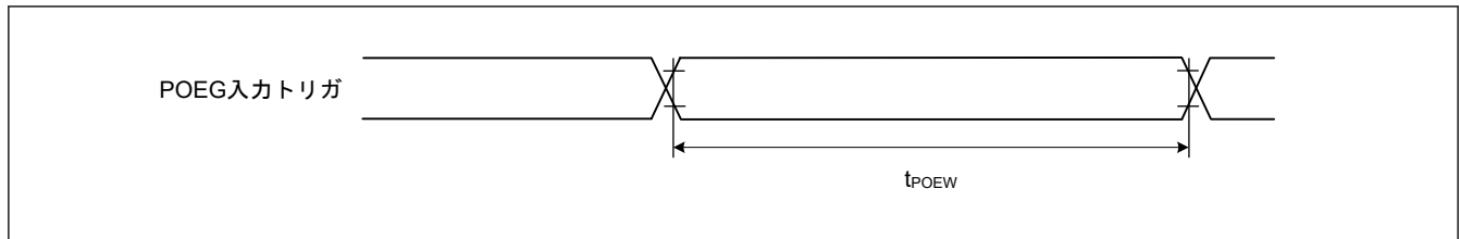
図 2.20 POEG 入力トリガタイミング
