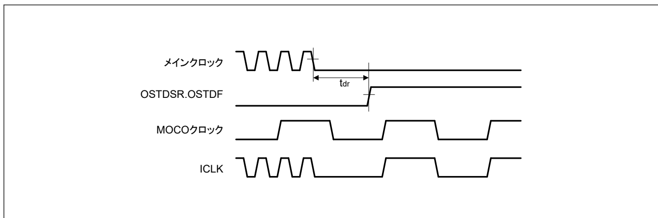
図 2.55 発振停止検出タイミング
