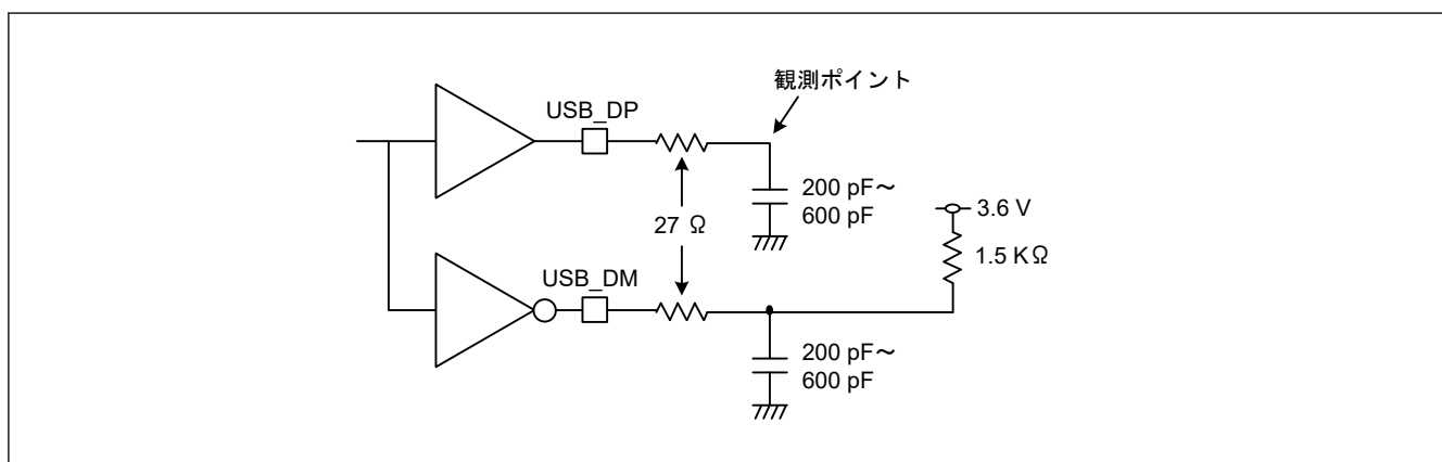
図 2.51 Low-speed モードにおける測定回路
