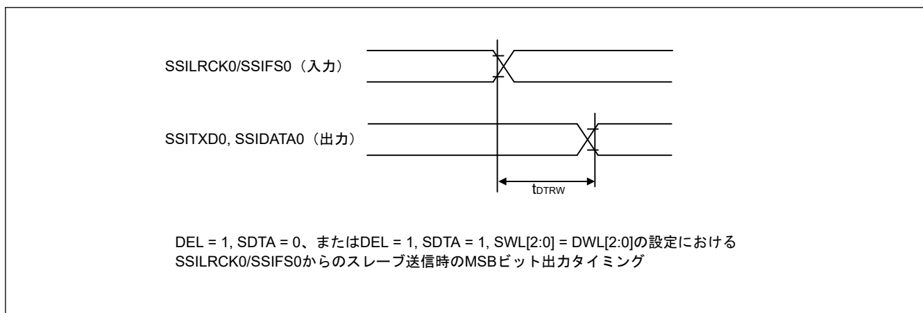
図 2.48 SSILRCK0/SSIFS0 変化時からの SSIE データ出力遅延
