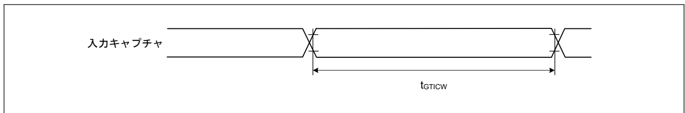
図 2.21 GPT インプットキャプチャタイミング
