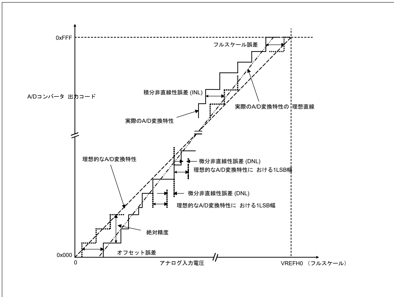
図 2.54 ADC12 特性用語の解説図
