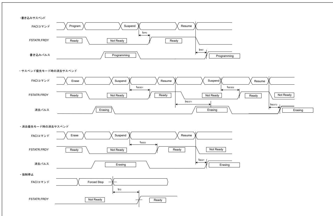
図 2.62 フラッシュメモリのプログラム/イレースのサスペンドタイミングと強制停止タイミング
