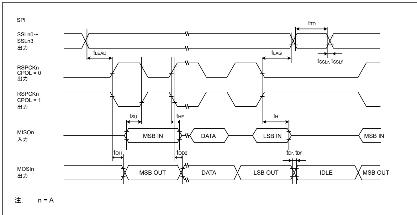
図 2.38 CPHA = 1 で、PCLKA/2 にビットレートが設定されている場合におけるマスタの RSPi タイミング
