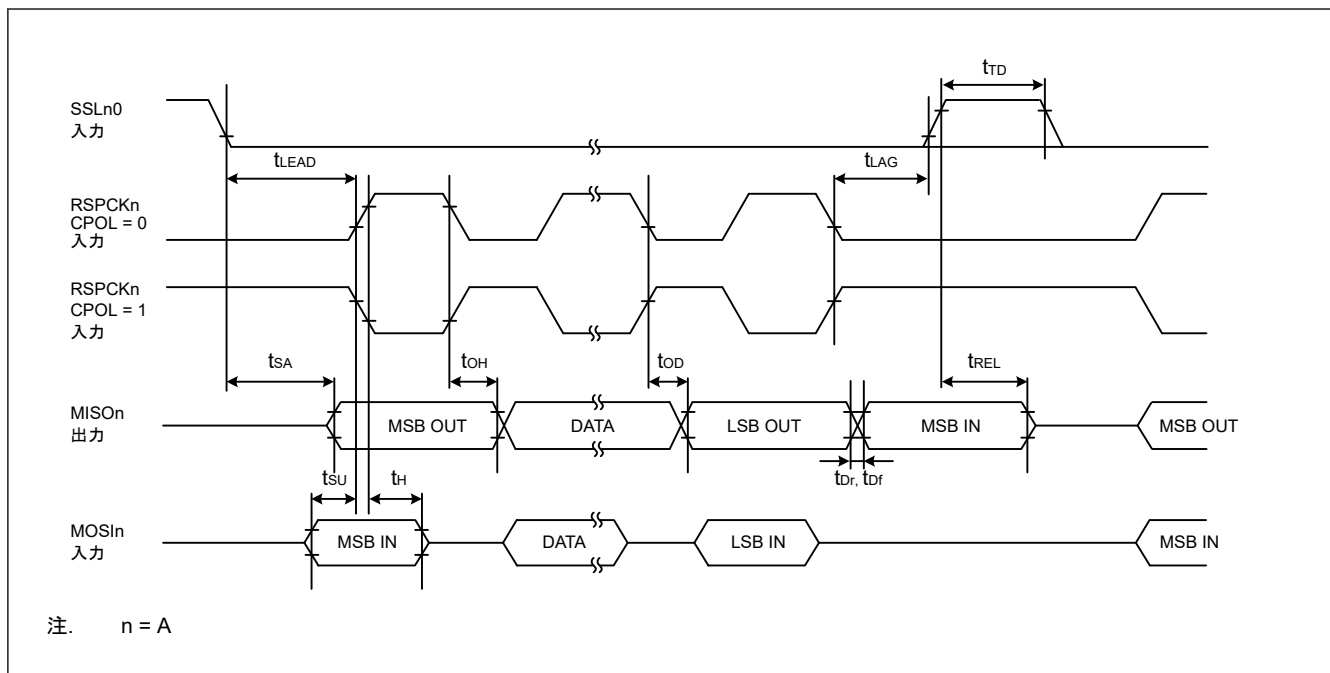
図 2.39 CPHA = 0 の場合におけるスレーブの RSPi タイミング
