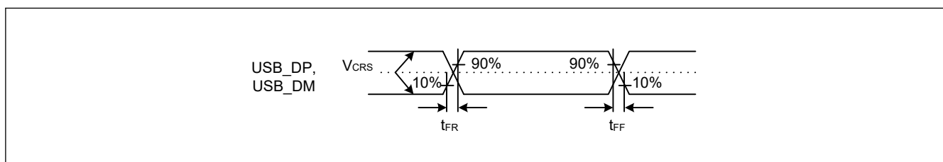
図 2.52 フルスピードモードにおける USB_DP、USB_DM の出カタイミング
