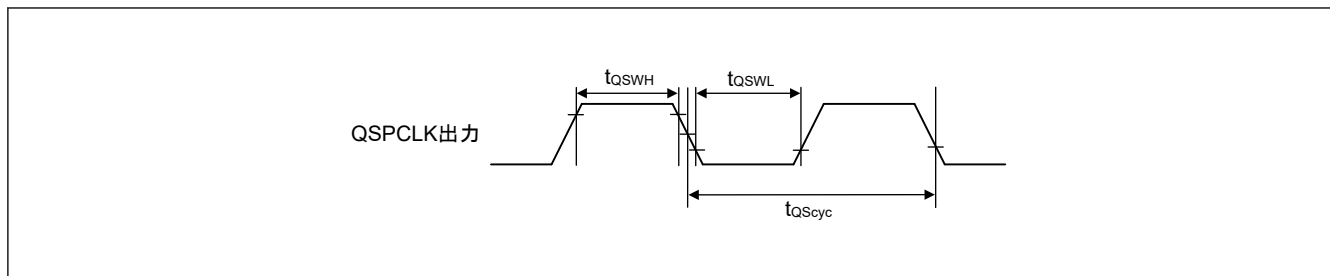
図 2.41 QSPI クロックタイミング
