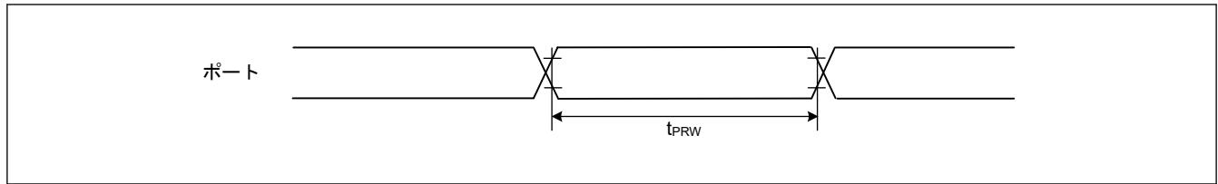
図 2.19 I/O ポート入力タイミング
