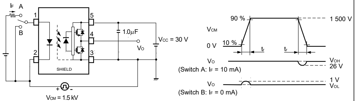
図9 CMR測定回路と波形
