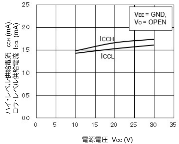
供給電流 vs. 電源電圧
