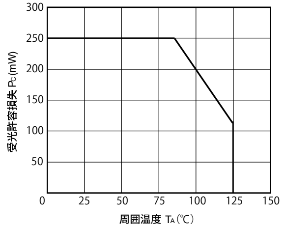
受光許容損失 vs. 周囲温度
