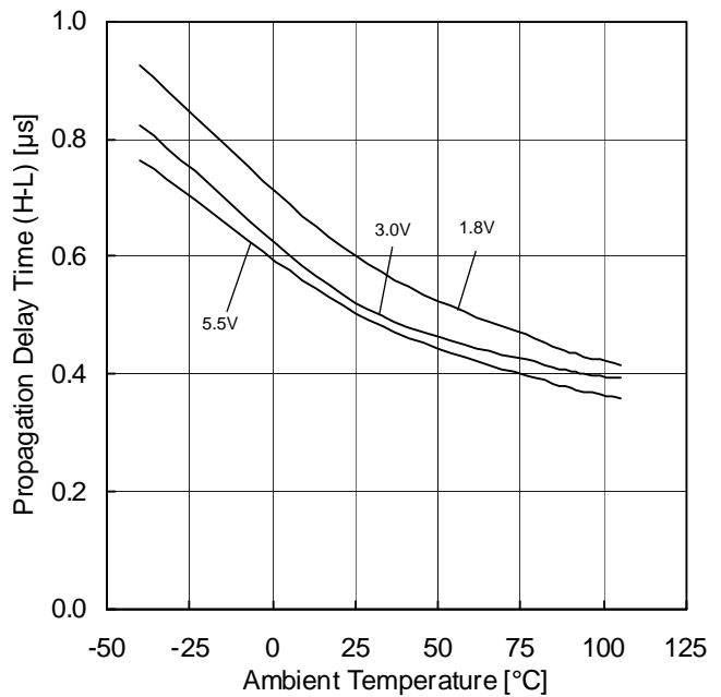
Figure 20. 立ち下がり伝播遅延時間—温度特性 ( R_L=10k\Omega , V_{RL}=3V , C_L=15pF I_N=1.5V , 100mV Overdrive)
