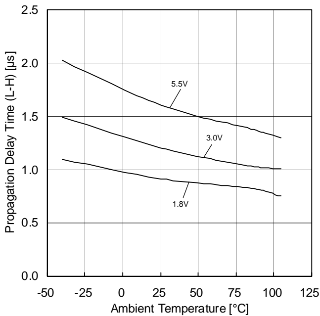
Figure 19. 立ち上がり伝播遅延時間—温度特性 ( R_L=10k\Omega , V_{RL}=3V , C_L=15pF I_N=1.5V , 100mV Overdrive)
