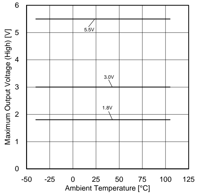
Figure 6. 最大出力電圧(High)－温度特性 ( R_L=10k\Omega , V_{RL}=V_{DD} )
