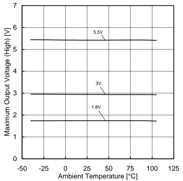
Figure 28. 最大出力電圧(High)－温度特性 ( R_L=10k\Omega )
