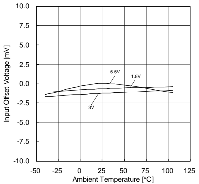
Figure 36. 入力オフセット電圧—温度特性 ( V_{ICM}=V_{DD} , E_K=-V_{DD}/2 )
