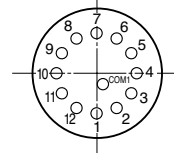
端子番号図
