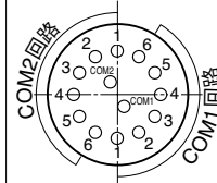
端子番号図
