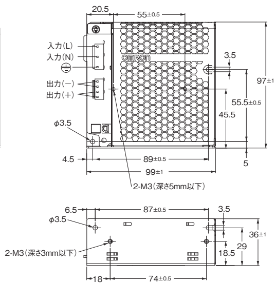
取り付け穴加工寸法
