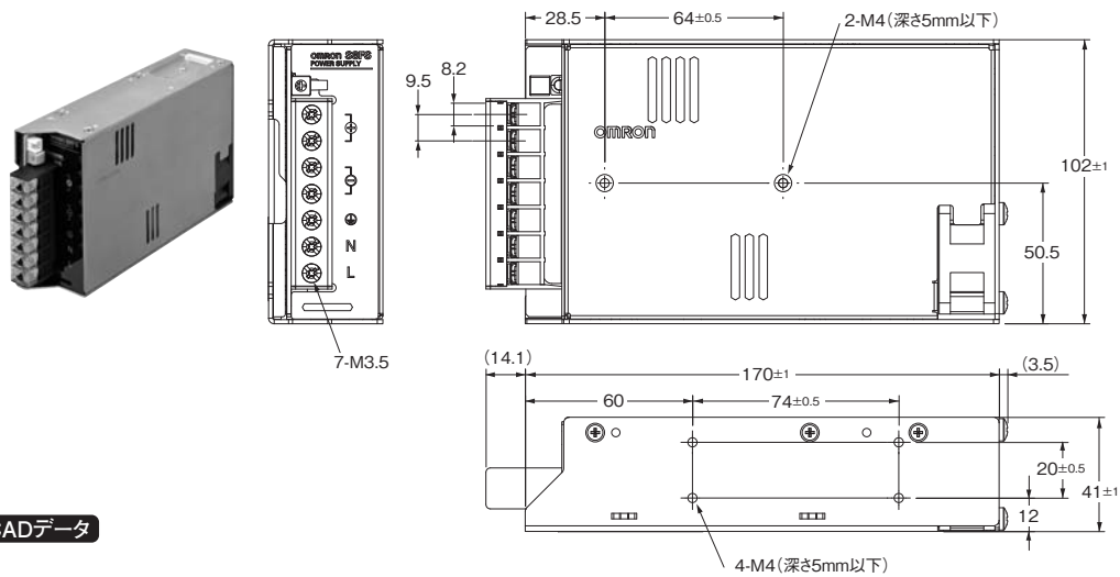
取り付け穴加工寸法
