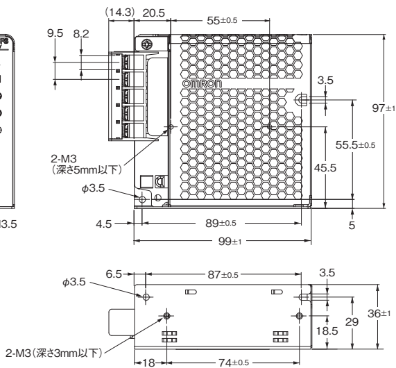
取り付け穴加工寸法
