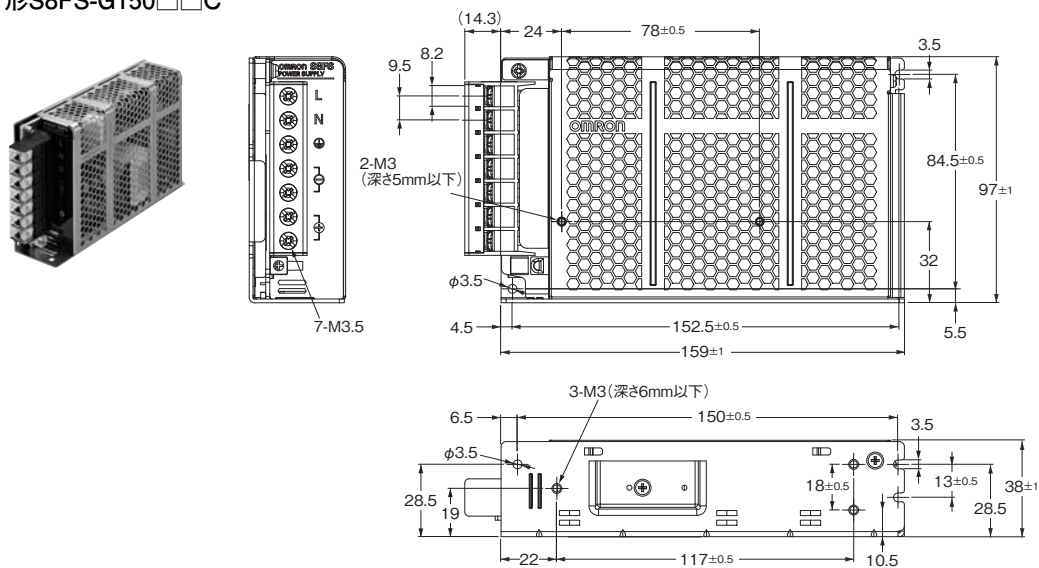
取り付け穴加工寸法
