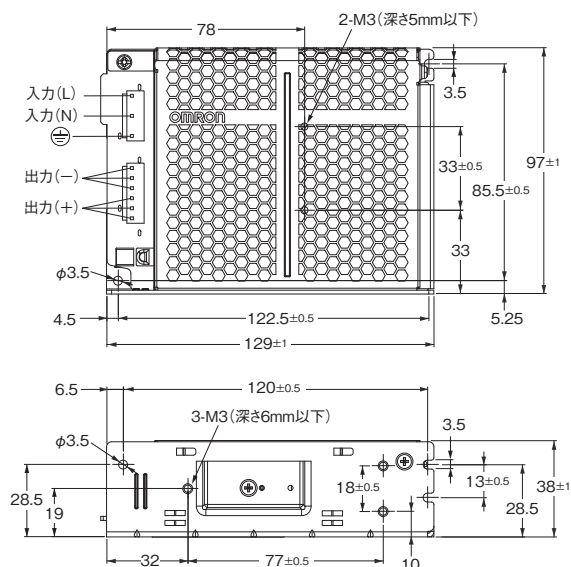
取りつけ穴加工寸法
