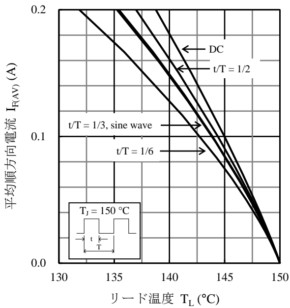
図2 I_{F(AV)} - T_L 代表特性 (2) ( V_R = 0\text{ V} )
