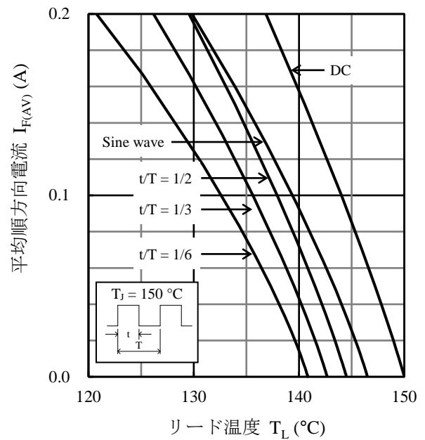
図3 I_{F(AV)} - T_L 代表特性 (2) ( V_R = 1000\text{ V} )
