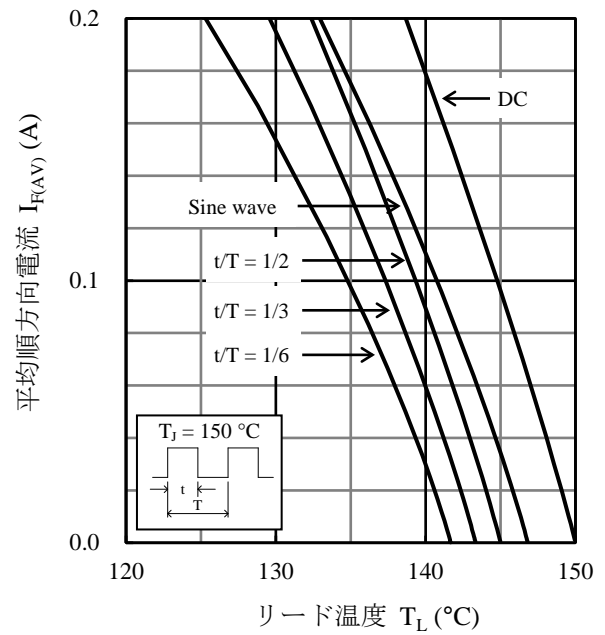
図3 I_{F(AV)} - T_L 代表特性 (2) ( V_R = 1000 V)
