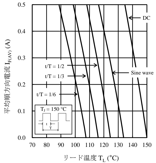
図3 I_{F(AV)} - T_L 代表特性 (2) ( V_R = 1500 \text{ V} )
