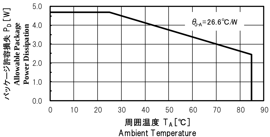
図 5-1 減定格図
