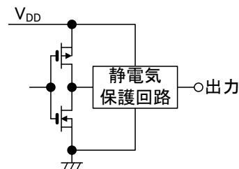
図 15-7 モニター出力端子内部等価回路
