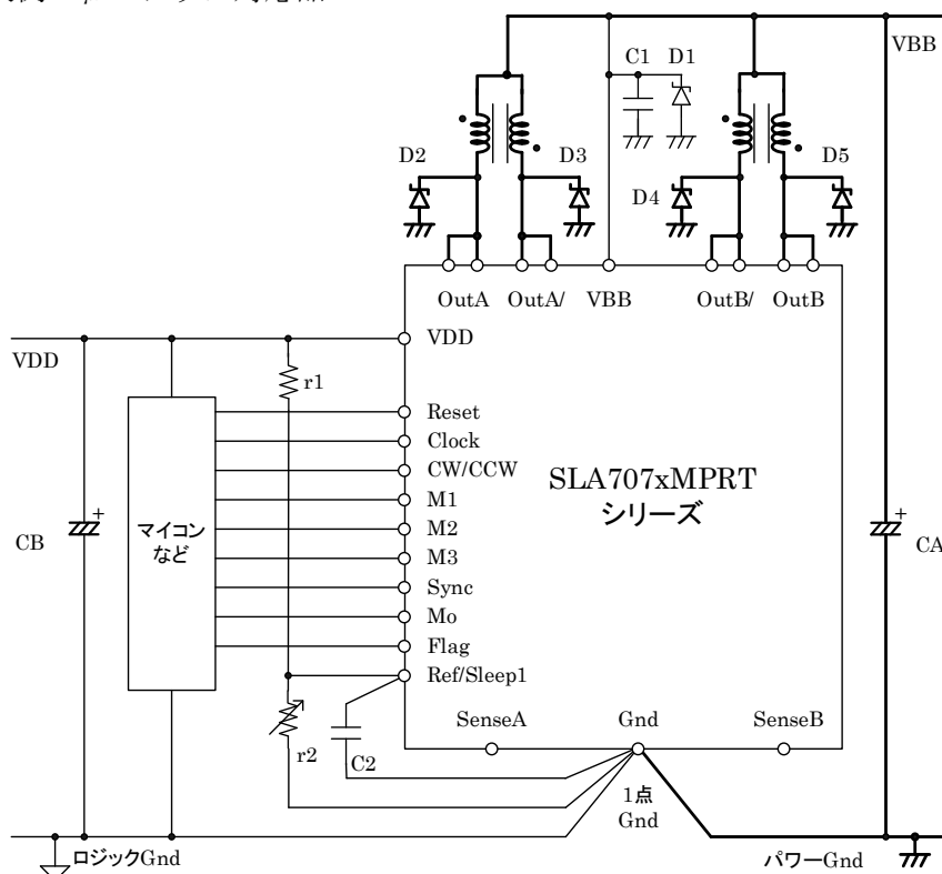
図 8-1 代表例： \mu ステップ対応品
