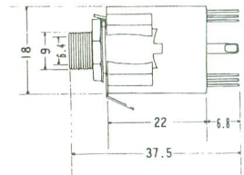
MJ-103 6.3φ3極オープンモールドジャック
