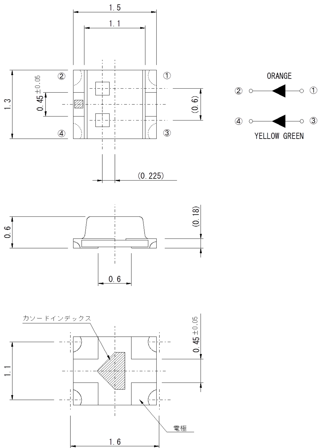
【図-1. 外形寸法図】
