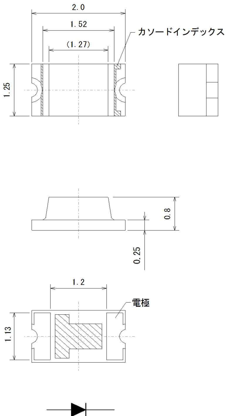
【図-1. 外形寸法図】
