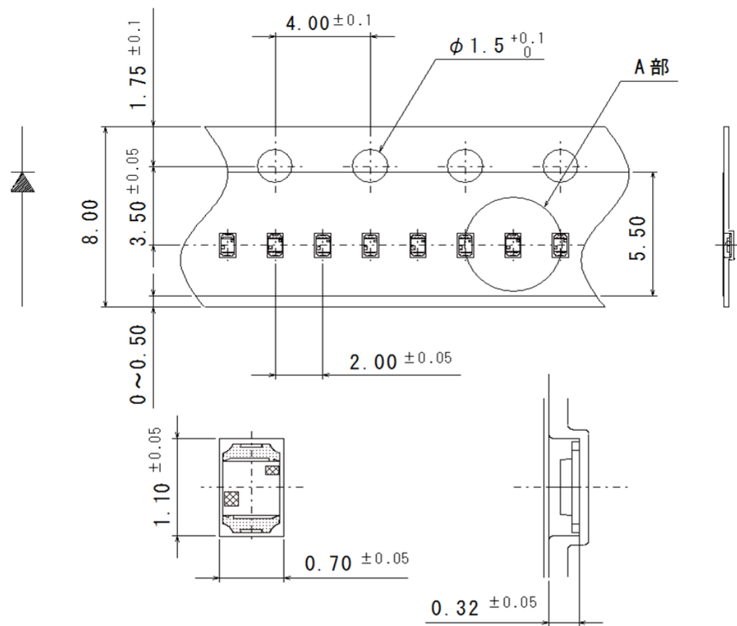
A部詳細
