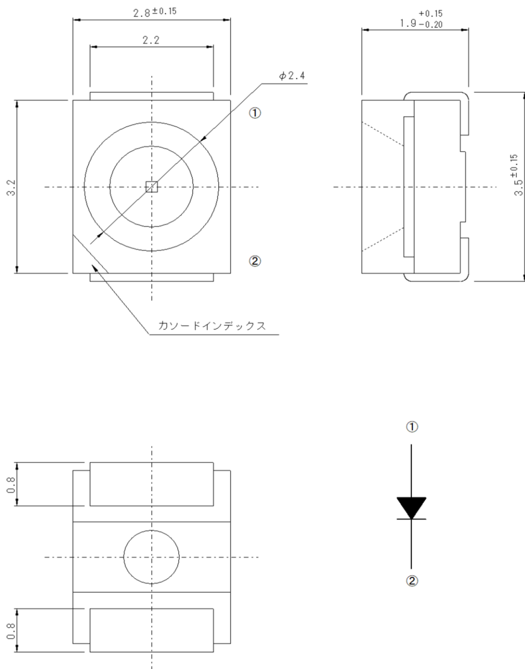
【図-1. 外形寸法図】
