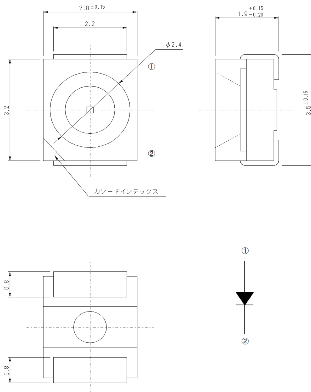
【図-1. 外形寸法図】
