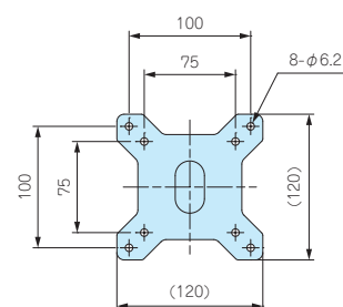
モニターブラケット寸法
