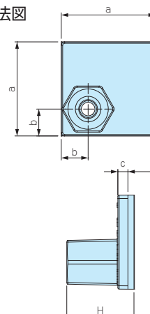
外観寸法図
