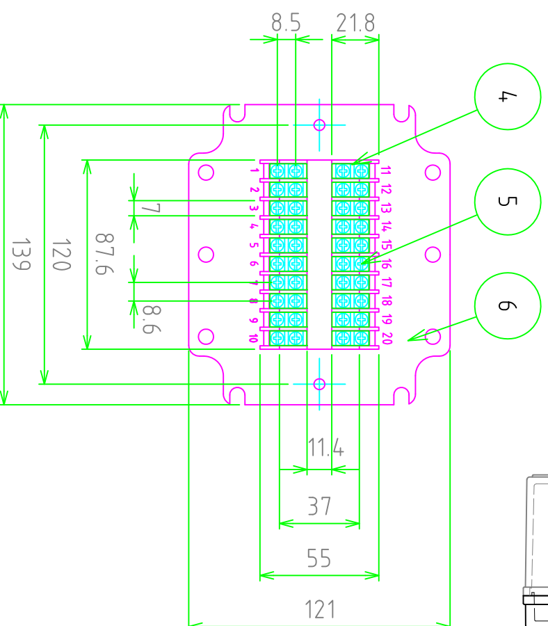
端子台詳細図
