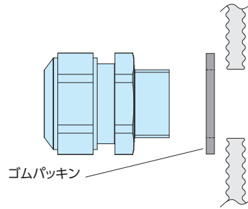
凹凸の大きい塗装品や鋳造品に取り付ける場合
