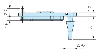
取付穴寸法図
