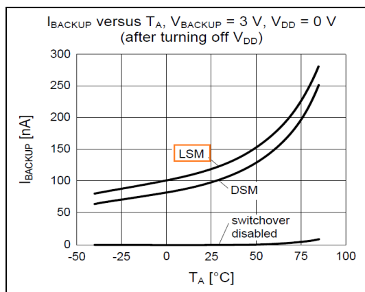
・Vbackup 動作時の Timekeeping状態での消費電流 ( "LSM" = レベル電源切替モード時の消費電流 )
