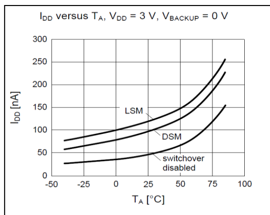
・Vdd 動作時の Timekeeping状態での消費電流
