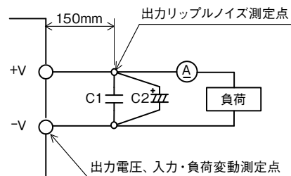
特性測定回路
