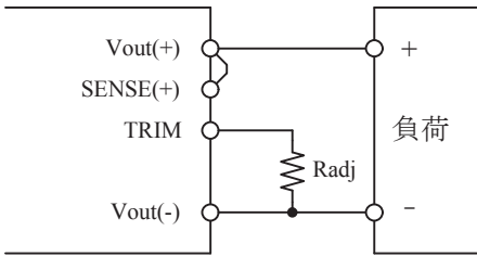
図6-1 出力可変用抵抗接続
