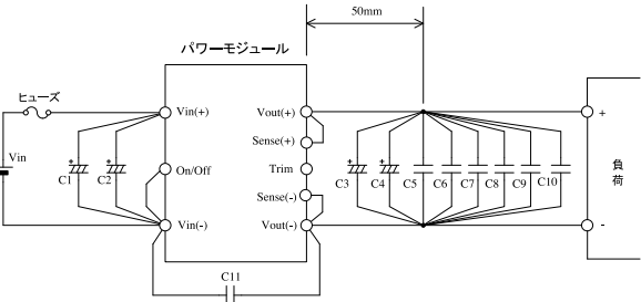
図1-1 基本的な接続
