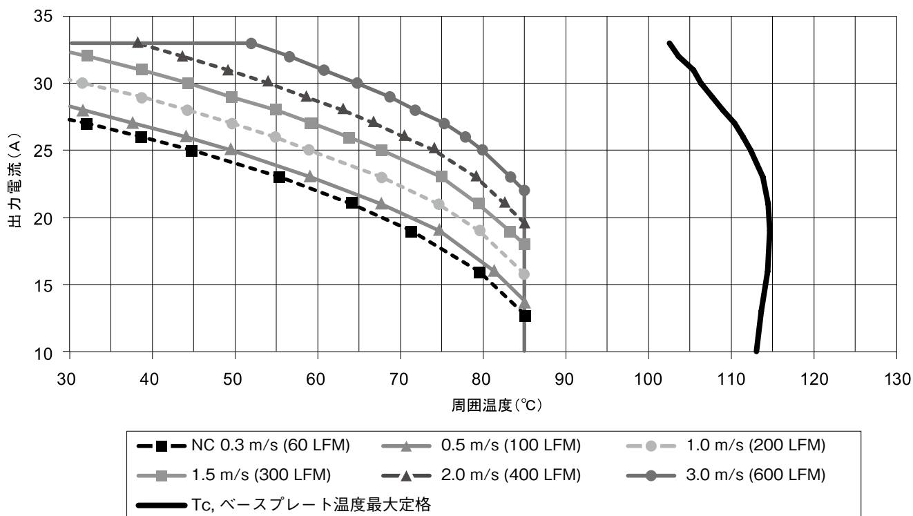
図A-13 iQG シリーズ 出力電流ディレーティングカーブ
