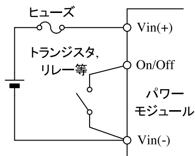
図11-1 On/Off 接続例
