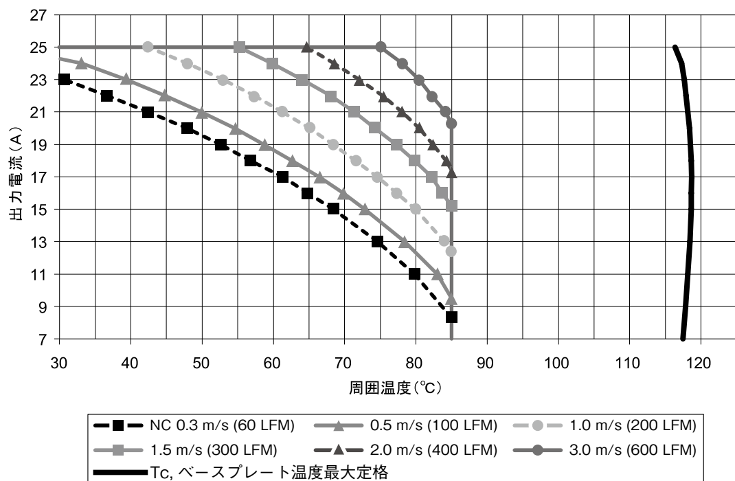
図A-12 iQL48025A120V-009-R 出力電流ディレーティングカーブ
