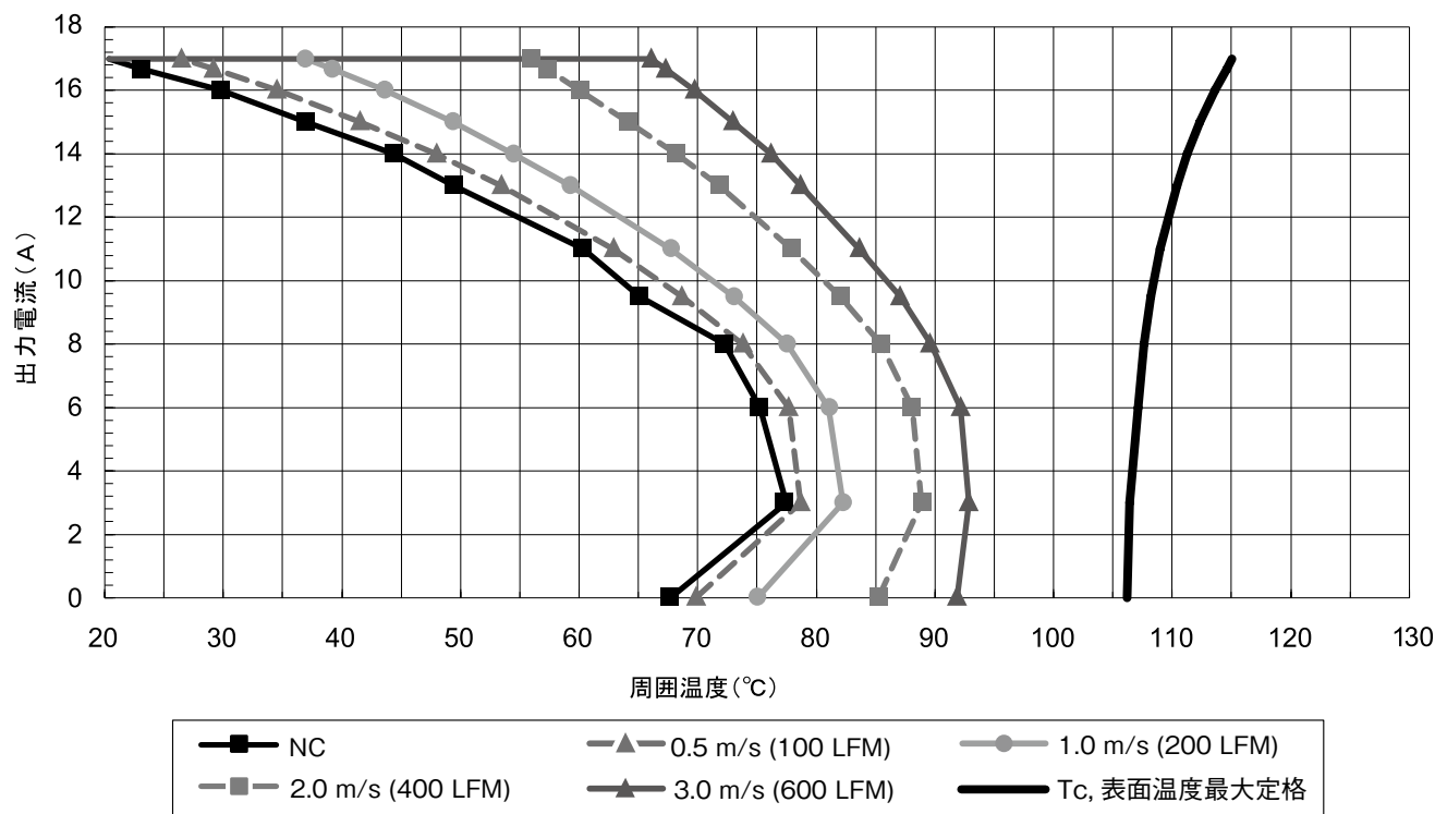
図A-6 iQE48017A120V-001-R 出力電流ディレーティングカーブ
