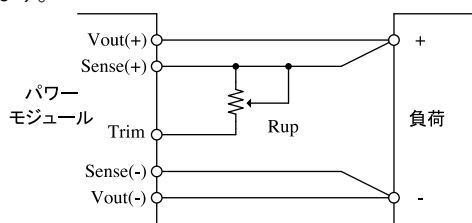
図6-3 可変抵抗接続(2)
