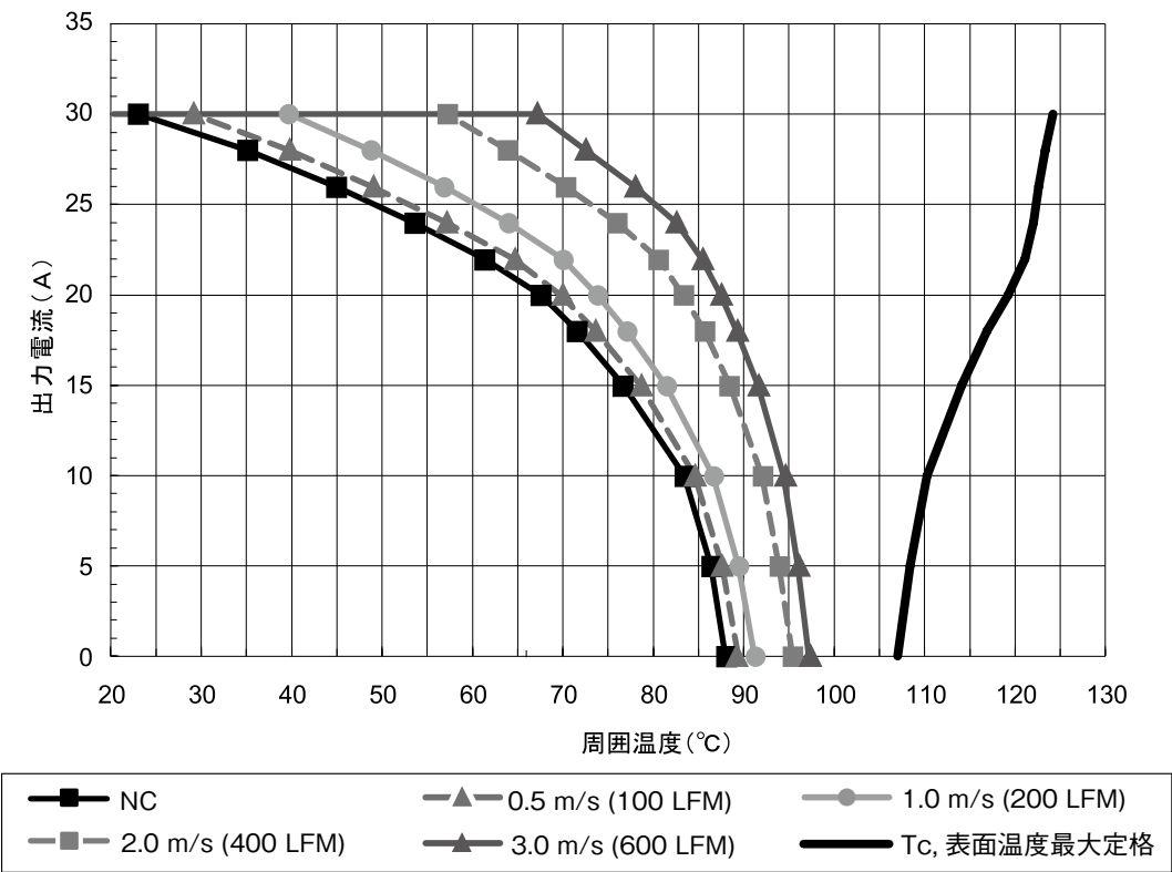
図A-7 iQE48030A050V-001-R 出力電流ディレーティングカーブ
