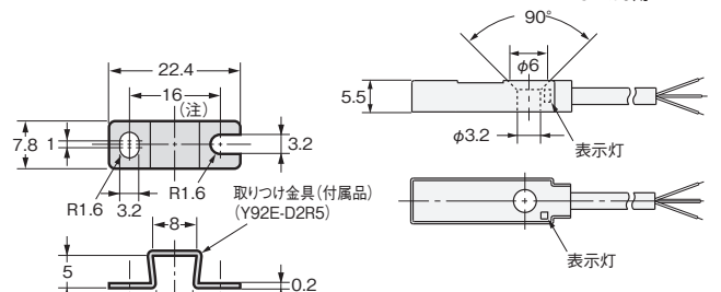
取り付け金具 (付属)
