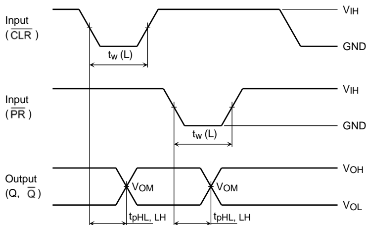
図 4 t_{pLH} , t_{pHL}
