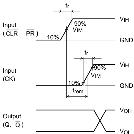
図 3 t_{rem}
