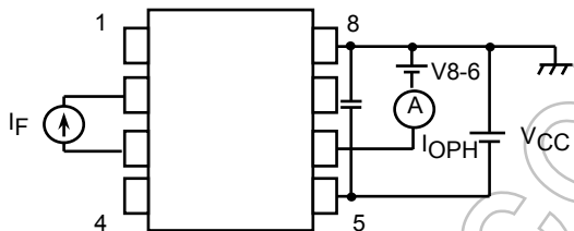
図1 I_{OPH} 測定回路図
