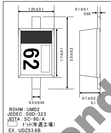
●外形寸法図 (Unit : mm)
