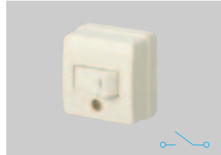
④WS3001W 標準価格 230円 税抜 10A角型タンブラスイッチE(片切) 10A300V ㊦ ④WS3002W(3路) 標準価格400円 税抜 もあります。
