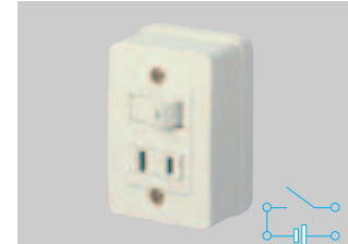
WS3901W 標準価格 700円 税抜 コンセント付タンブラスイッチ(ハイ角連用) スイッチ10A300V コンセント15A125V
