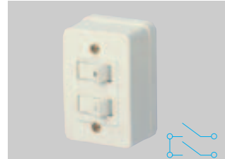
WS3900W 標準価格 760円 税抜 2連タンブラスイッチ(ハイ角連用) 10A300V
