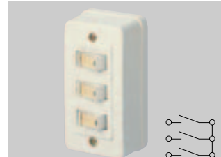
WS3910W 標準価格 1,300円 税抜 3連タンブラスイッチ(カード付) 10A300V
