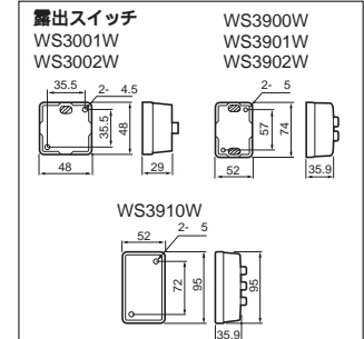
WS3901W 標準価格 700円 税抜 コンセント付タンブラスイッチ(ハイ角連用) スイッチ10A300V コンセント15A125V
